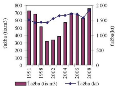
Graf 171. Vývoj v ťažbe vápencov a cementárskych surovín
