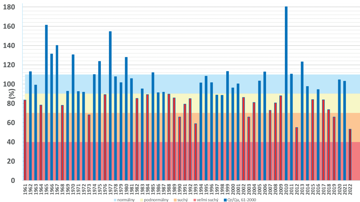
Graf 072 | Vývoj priemernej ročnej vodnosti roka povrchových tokov v SR
