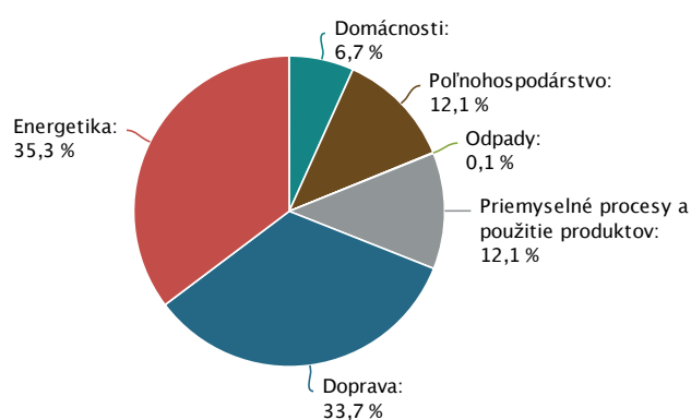
Graf 075 | Podiel emisií NO x podľa sektorov (2021)
