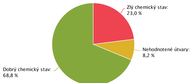
Graf 009 | Chemický stav útvarov podzemnej vody vyhodnotený v rámci tretieho cyklu plánov manažmentu povodí (Podiel plochy)
