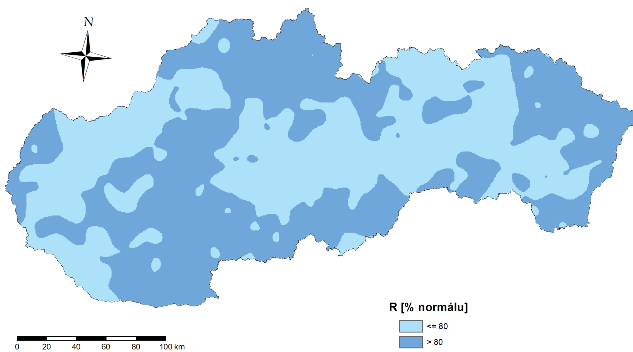
Mapa 016 | Percento normálu (1991 – 2020) ročných úhrnov zrážok za rok 2022
