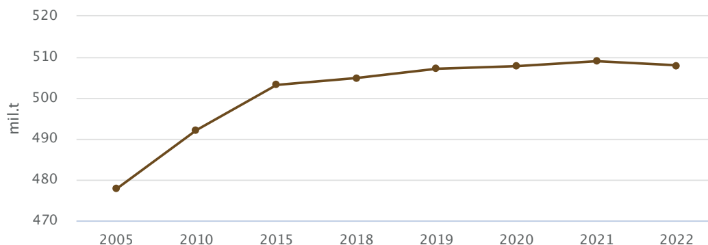
Graf 045 | Vývoj zásoby uhlíka v lesných ekosystémoch
