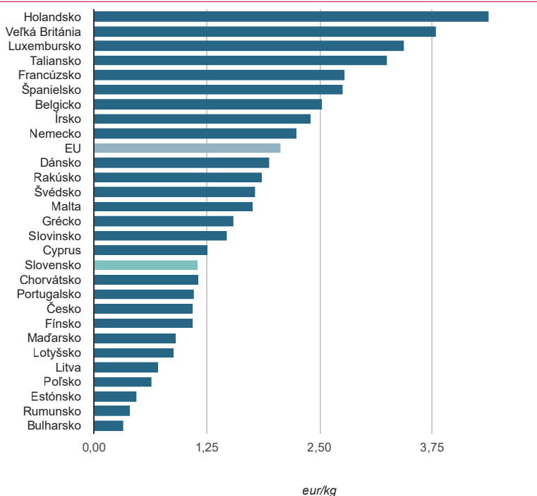
Graf 129 I Medzinárodné porovnanie produktivity zdrojov (2017)
