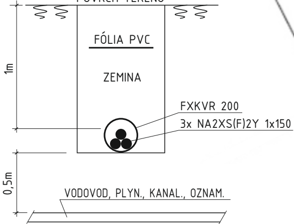
REZ ULOŽENÍM VN KÁBLOV V ZEMY
