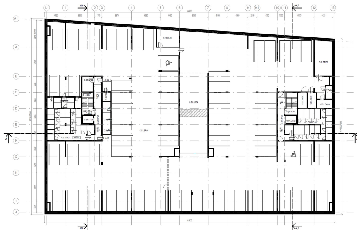
Obr. 4 pôdorys 1.PP
