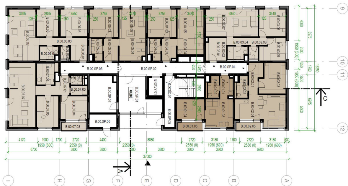
Obr. 9 pôdorys 1.NP, 01/SO1 - Bytový dom B
