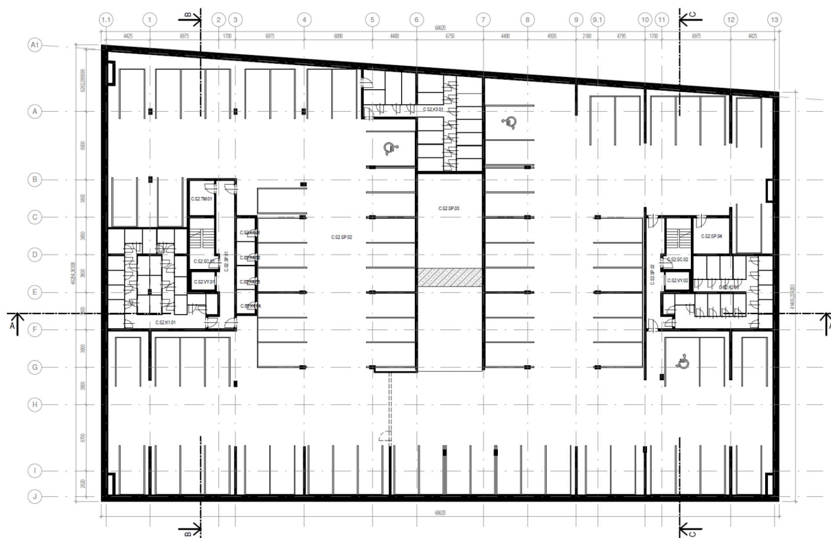
Obr. 3 pôdorys 2.PP
