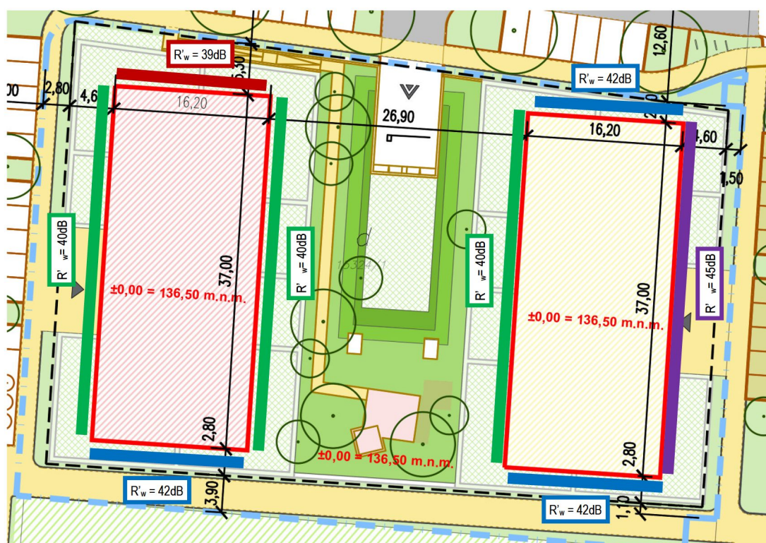
Obr. 30 pôdorys strechy, minimálne požadované hodnoty zvukovej izolácie R'_w obvodových plášťov. Uvedené hodnoty sú hodnotami požadovanými pre obvodový plášť ako celok, vrátane konštrukcií výplní otvorov
