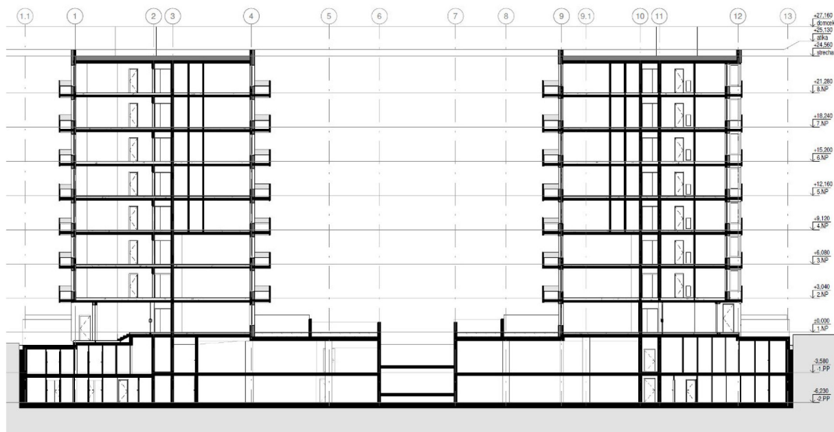
Obr. 12 rez objektom 01/SO1
