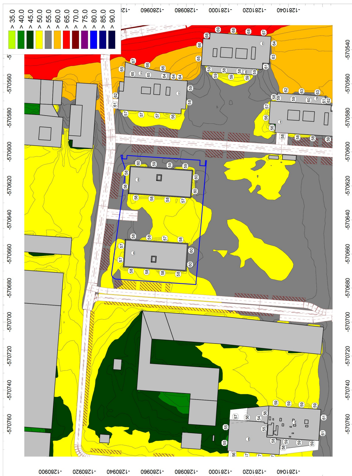
Obr. 25 hluková záťaž vypočítaná vo výške 1,5 m nad terénom, pre nočný referenčný časový interval a hodnoty ekvivalentných hladín A zvuku pred fasádami najbližších chránených objektov, delenie pásiem po 5 dB
