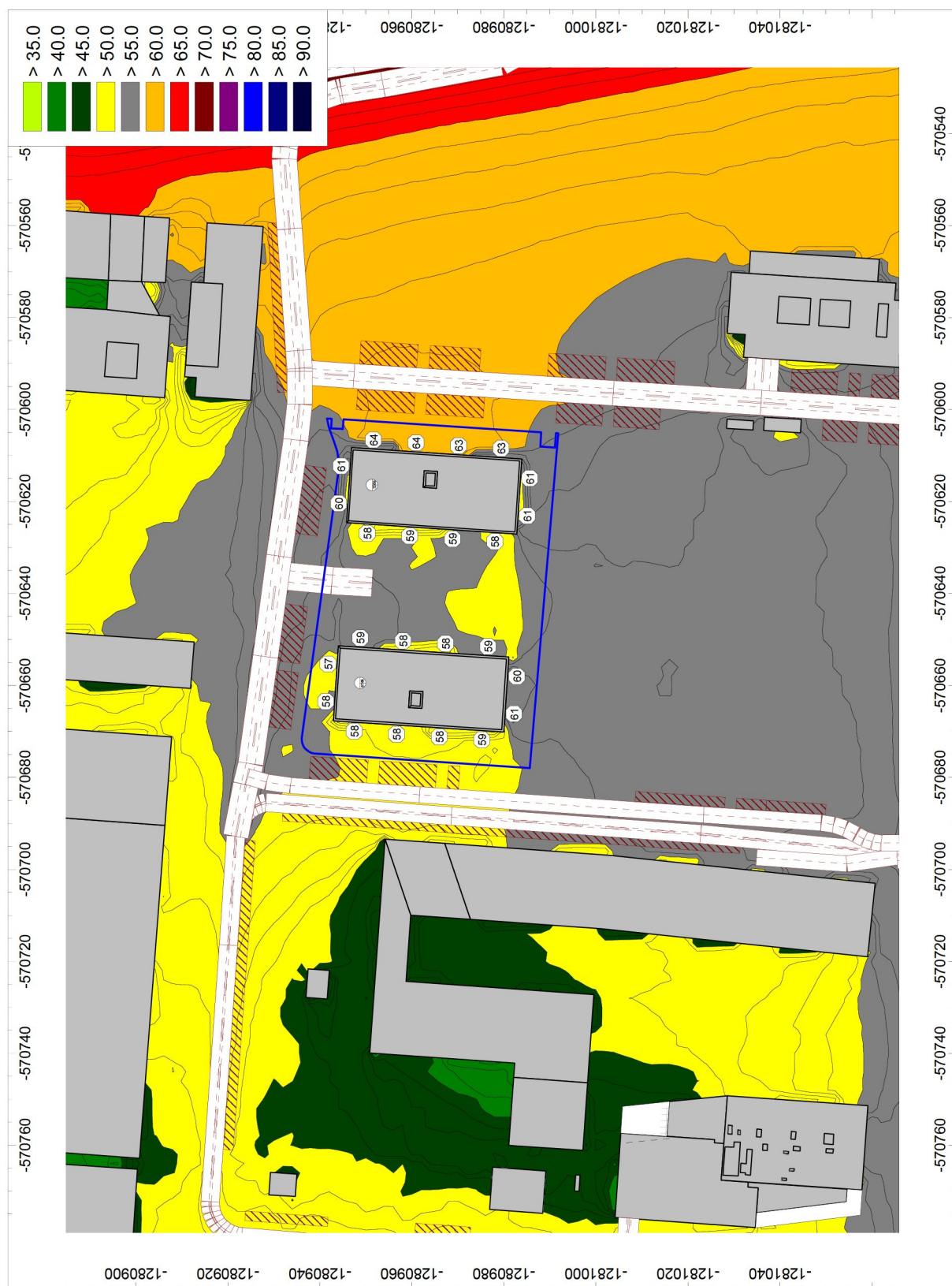
Obr. 29 hluková záťaž vypočítaná vo výške 1,5 m nad terénom, pre nočný referenčný časový interval a hodnoty ekvivalentných hladín A zvuku pred fasádami najbližších chránených objektov, delenie pásiem po 5 dB
