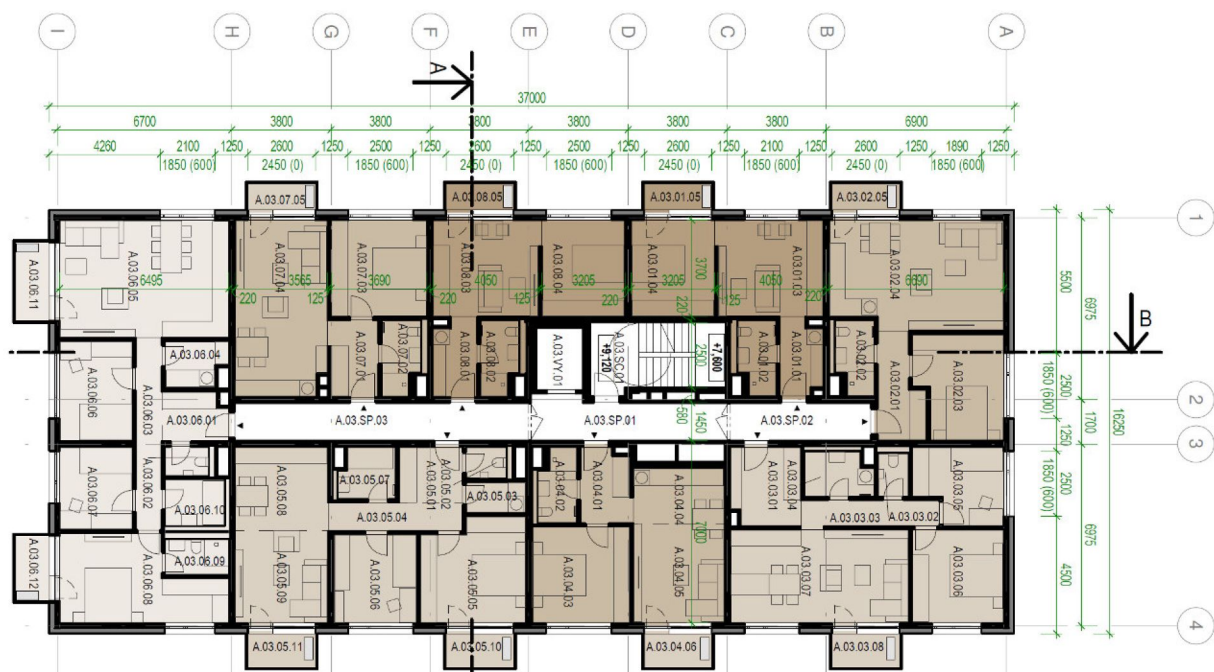
Obr. 7 pôdorys 4. – 8.NP, 01/SO1 - Bytový dom A
