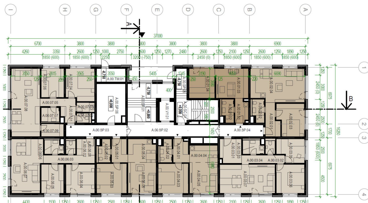
Obr. 5 pôdorys 1.NP, 01/SO1 - Bytový dom A
