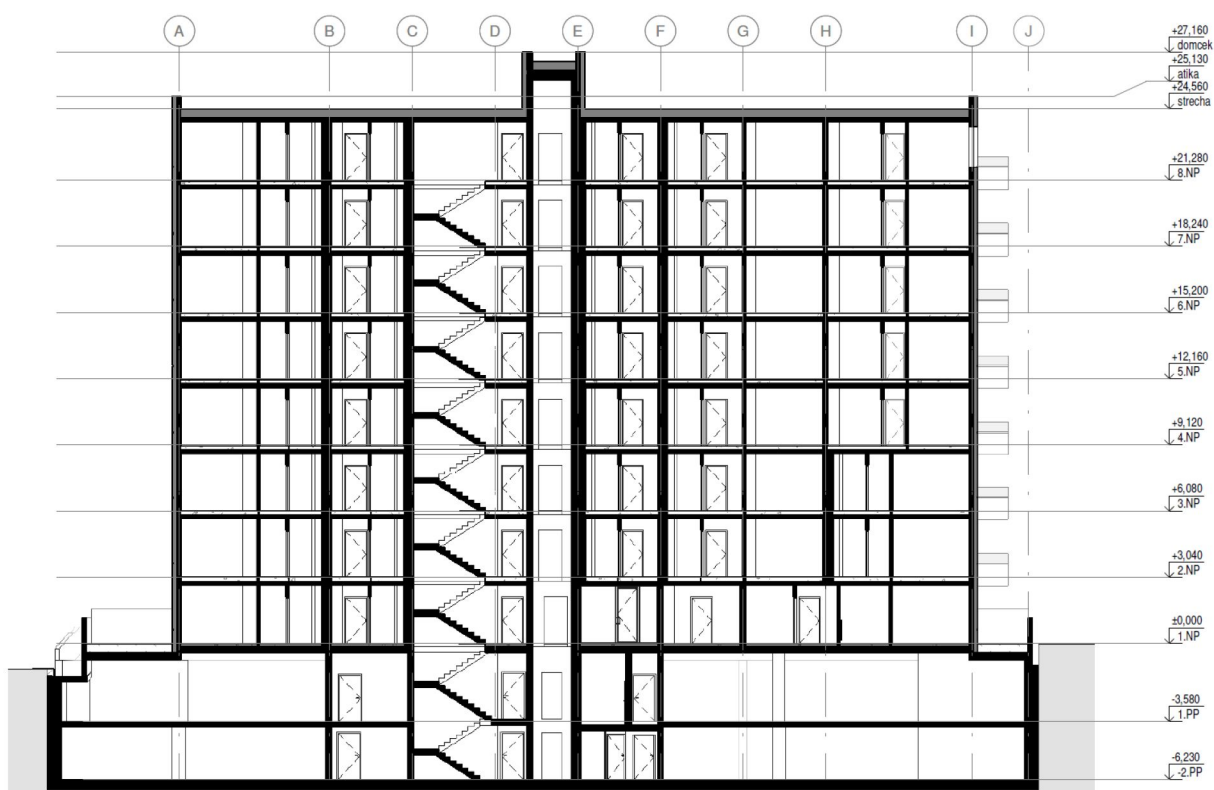
Obr. 8 rez objektom 01/SO1 - Bytový dom A
