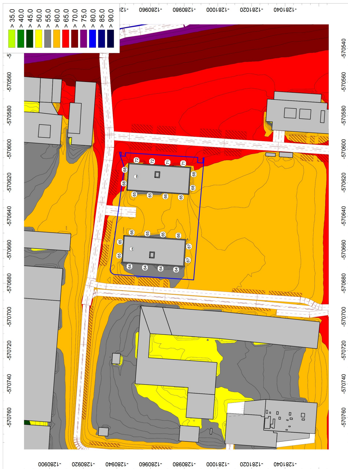
Obr. 27 hluková záťaž vypočítaná vo výške 1,5 m nad terénom, pre denný referenčný časový interval a hodnoty ekvivalentných hladín A zvuku pred fasádami najbližších chránených objektov, delenie pásiem po 5 dB
