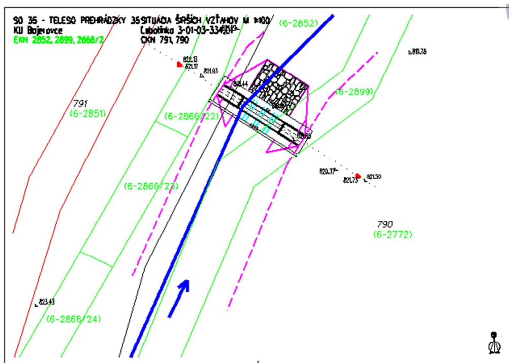
Celková situácia umiestnenia SO 35
