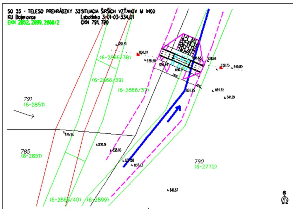
Celková situácia umiestnenia SO 33
