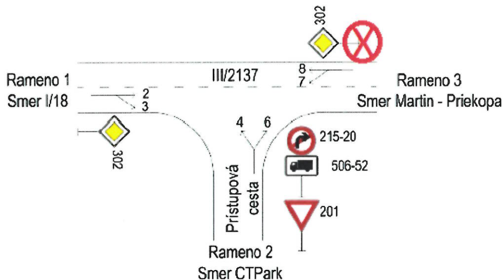
Obrázok 2-2 Schéma posudzovanej križovatky
