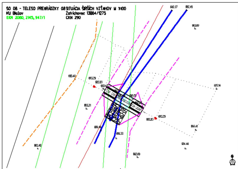
Celková situácia umiestnenia SO 08
