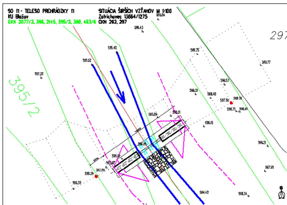
Súradnice polohy stavebného zámeru SO 11
