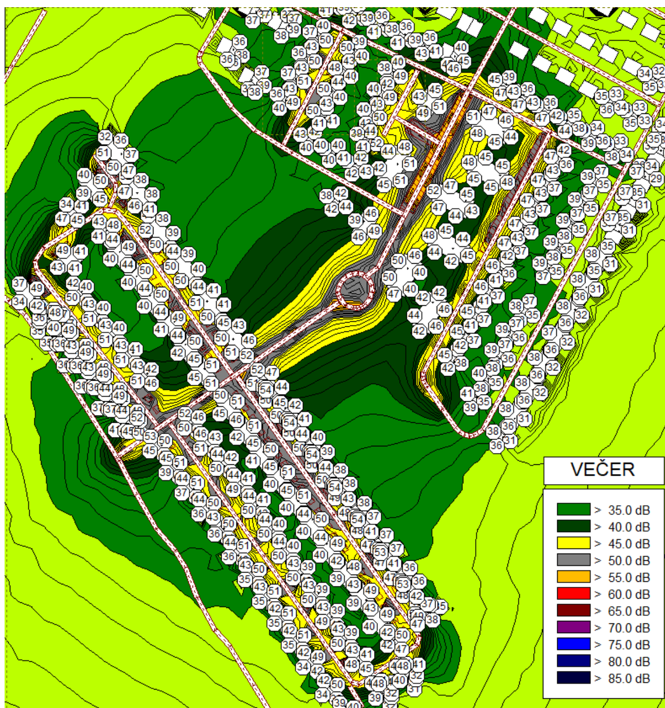
Obrázok 15 Plošná hluková záťaž spôsobená statickou dopravou vypočítaná vo výške 1,5 m nad terénom a najvyššie hodnoty L_{Aeq} 2 m pred fasádami posudzovaných objektov a okolitých budov pre referenčný časový interval VEČER
