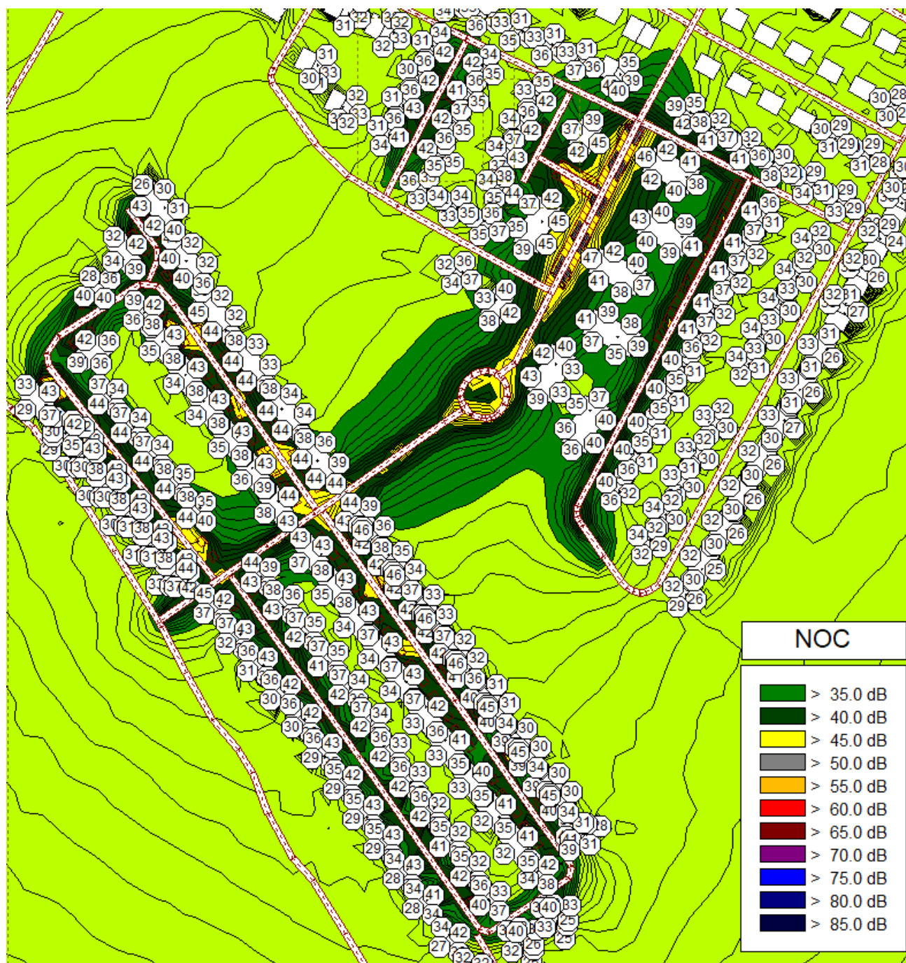
Obrázok 16 Plošná hluková záťaž spôsobená statickou dopravou vypočítaná vo výške 1,5 m nad terénom a najvyššie hodnoty L_{Aeq} 2 m pred fasádami posudzovaných objektov a okolitých budov pre referenčný časový interval NOC
