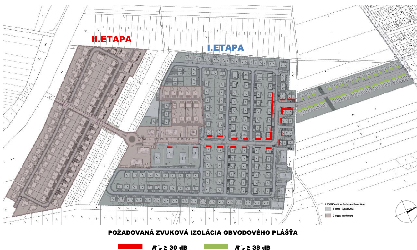
Obrázok 23 Požadovaná minimálna zvukovej izolácie obvodového plášťa rodinných a bytových domov I. etapy
