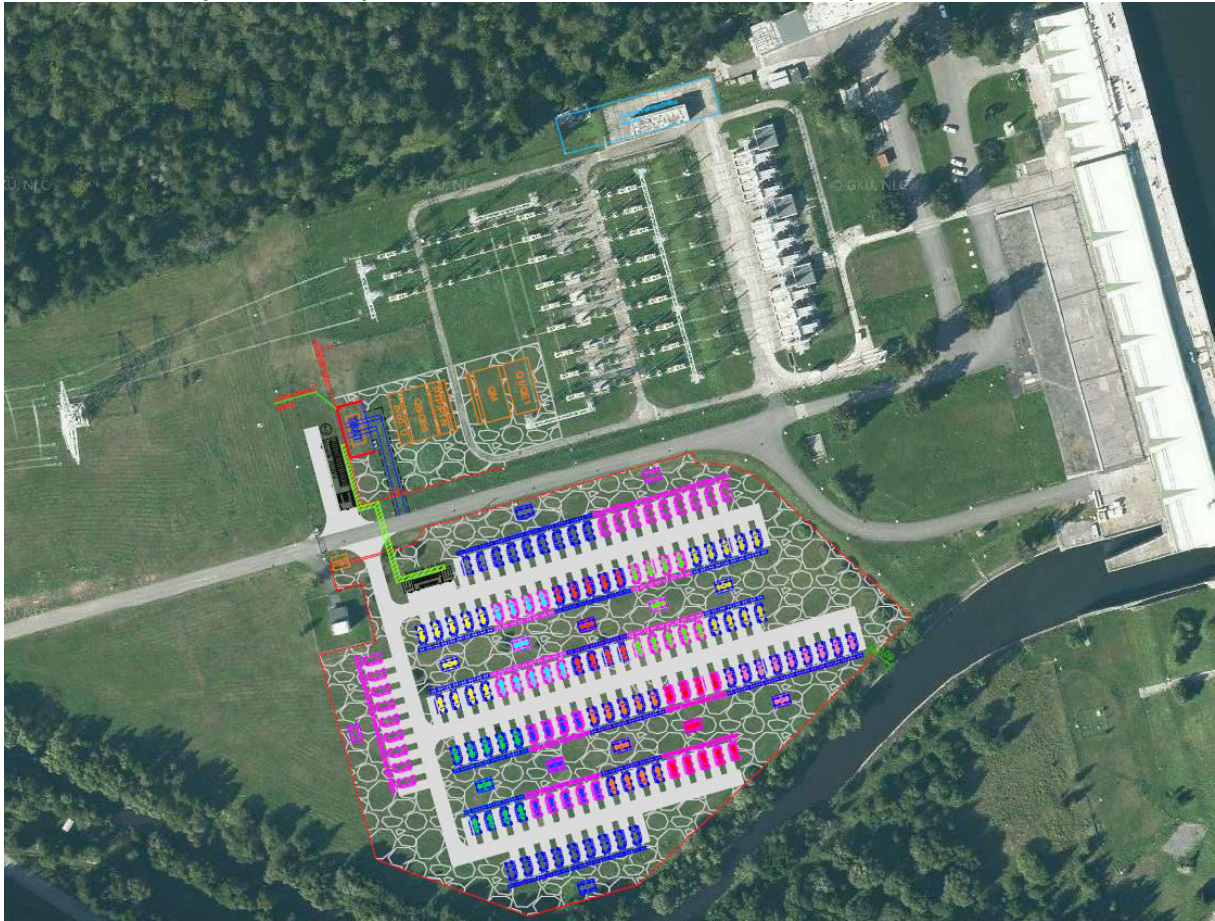
Obr. 6 Návrh dispozičného usporiadania BESS a R400 kV na PVE Čierny Váh
