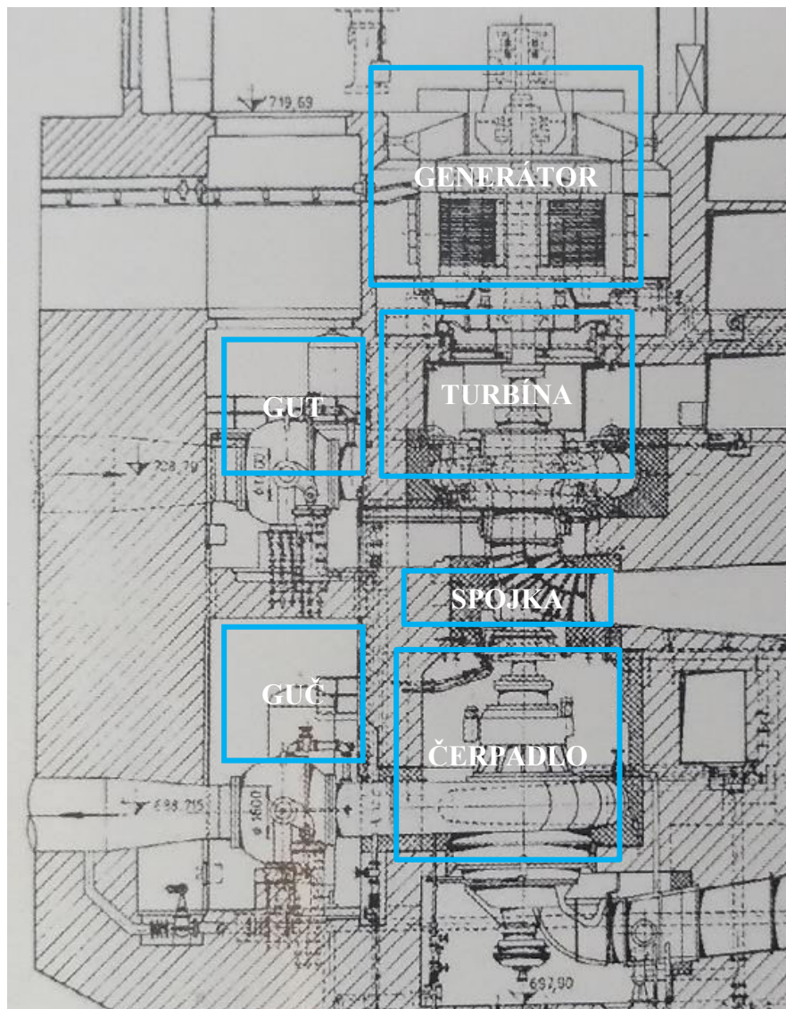
Obr. 4 Pohľad na modernizované časti TG1 (TG2)
