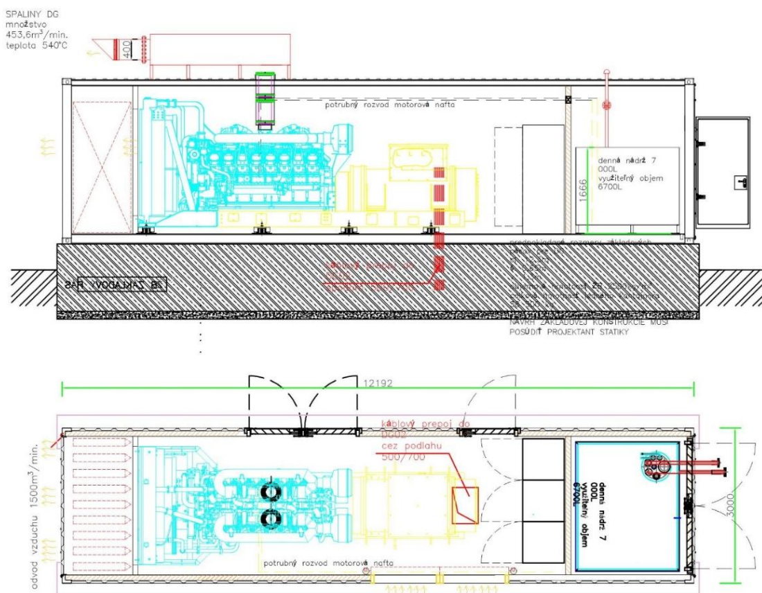
Obrázok č. 3 Technologický kontajner [D1]
