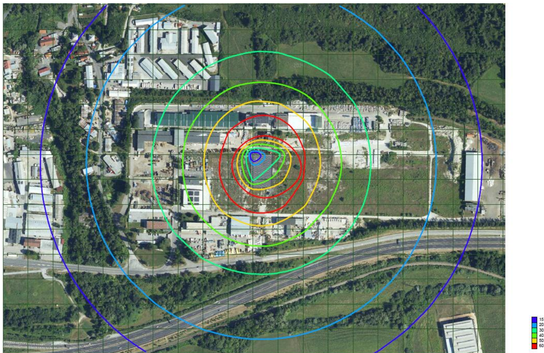
Príloha č. 6 Maximálne krátkodobé koncentrácie CO [ \mu\text{g}/\text{m}^3 ] – izočiary rozptylu emisií ZL zo zdrojov znečisťovania ovzdušia
