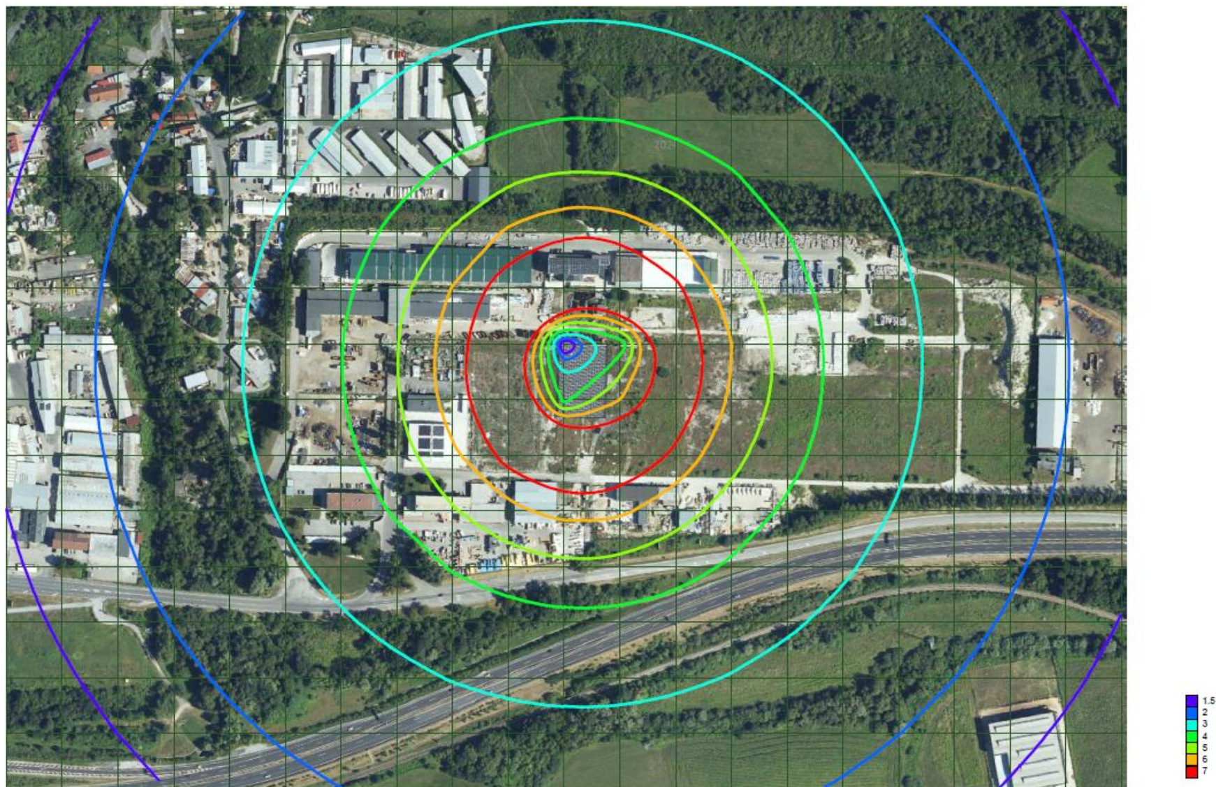
Príloha č. 3 Maximálne krátkodobé koncentrácie PM_{2,5} [ \mu g/m^3 ] – izočiare rozptylu emisií ZL zo zdrojov znečisťovania ovzdušia
