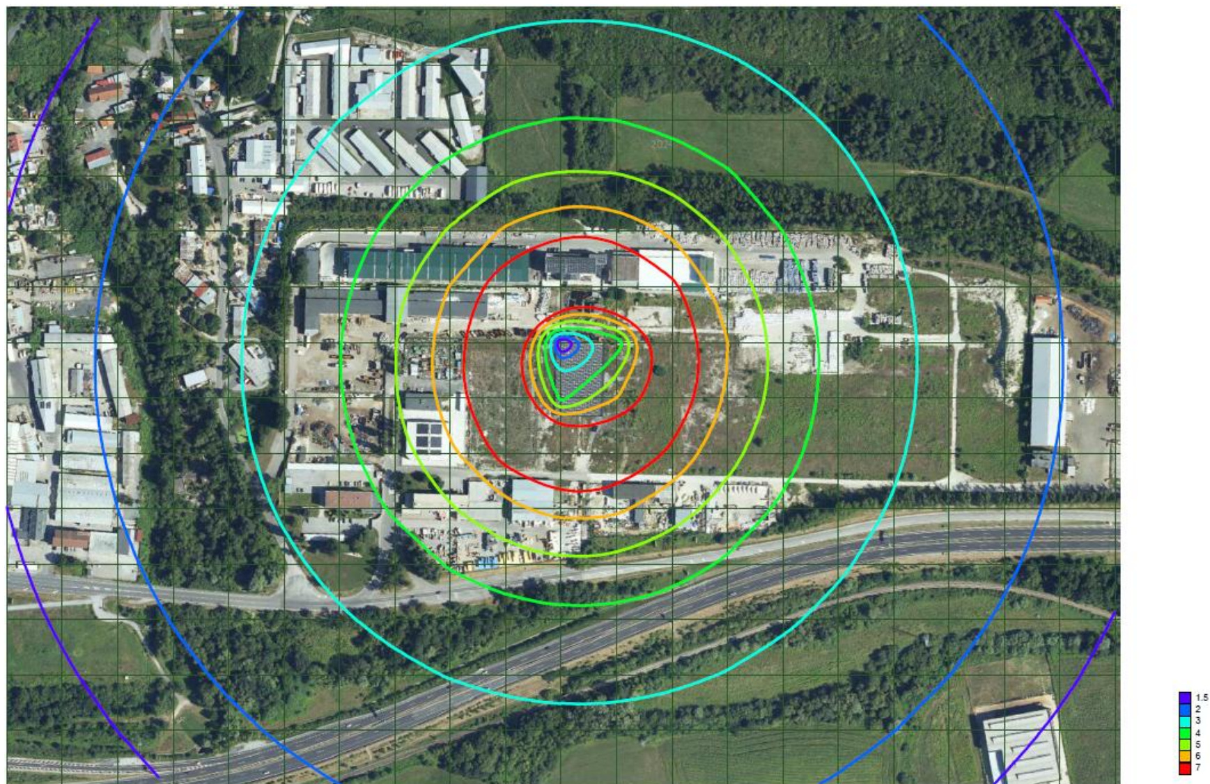
Príloha č. 4 Maximálne krátkodobé koncentrácie \text{SO}_2 [ \mu\text{g}/\text{m}^3 ] – izočiare rozptylu emisií ZL zo zdrojov znečisťovania ovzdušia
