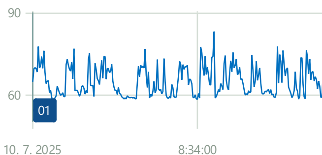
GRAF 9 Zobrazenie časového priebehu ekvivalentných hladín L_{Aeq,T} v meracom bode M9 – meranie vyloženia tovaru z nákladného vozidla
