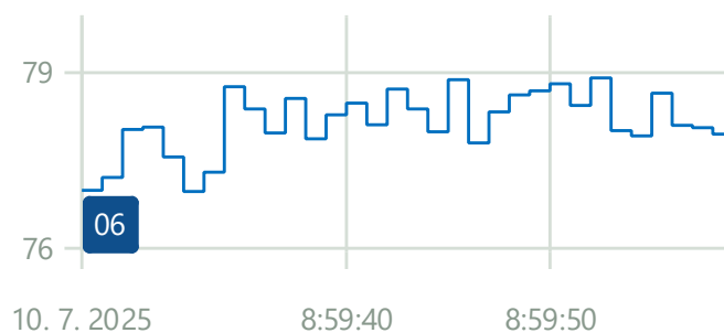
GRAF 6 Zobrazenie časového priebehu ekvivalentných hladín L_{Aeq,T} v meracom bode M6 – meranie chladiacej jednotky
