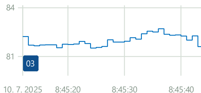
GRAF 3 Zobrazenie časového priebehu ekvivalentných hladín L_{Aeq,T} v meracom bode M3 – meranie výdychu na fasáde
