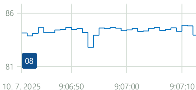
GRAF 8 Zobrazenie časového priebehu ekvivalentných hladín L_{Aeq,T} v meracom bode M8 – meranie čerpadla
