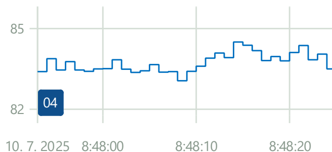
GRAF 4 Zobrazenie časového priebehu ekvivalentných hladín L_{Aeq,T} v meracom bode M4 – meranie výdychu na fasáde
