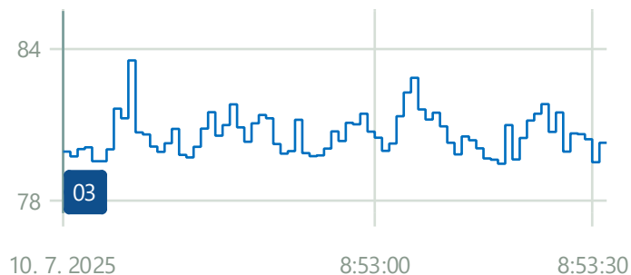
GRAF 11 Zobrazenie časového priebehu ekvivalentných hladín L_{Aeq,T} v meracom bode M11 – meranie čerpadla
