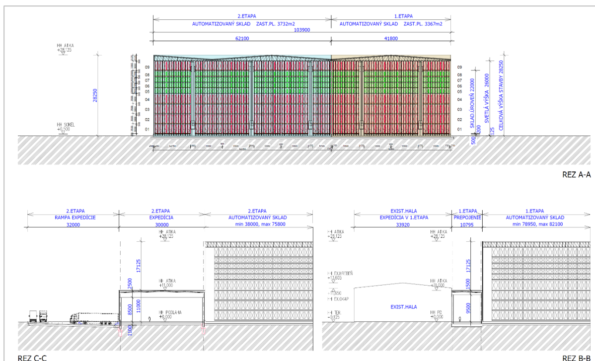
OBR. 8 Rezy – navrhovaný automatizovaný sklad plastových výrobkov
