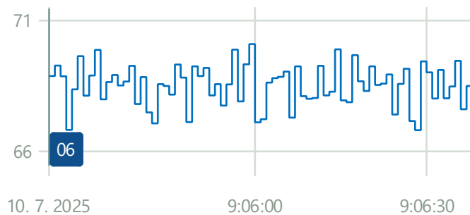
GRAF 13 Zobrazenie časového priebehu ekvivalentných hladín L_{Aeq,T} v meracom bode M13 – meranie čerpadla
