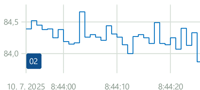
GRAF 2 Zobrazenie časového priebehu ekvivalentných hladín L_{Aeq,T} v meracom bode M2 – meranie výdychu na fasáde
