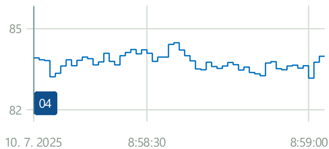
GRAF 12 Zobrazenie časového priebehu ekvivalentných hladín L_{Aeq,T} v meracom bode M12 – meranie čerpadla
