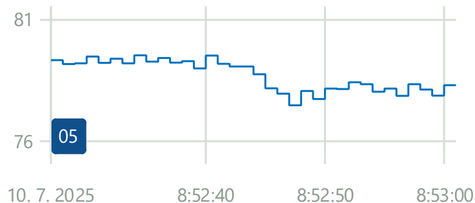
GRAF 5 Zobrazenie časového priebehu ekvivalentných hladín L_{Aeq,T} v meracom bode M5 – meranie čerpadla
