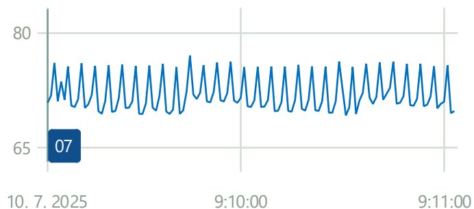
GRAF 14 Zobrazenie časového priebehu ekvivalentných hladín L_{Aeq,T} v meracom bode M14 – meranie hluku z otvorenej brány výrobnjej haly
