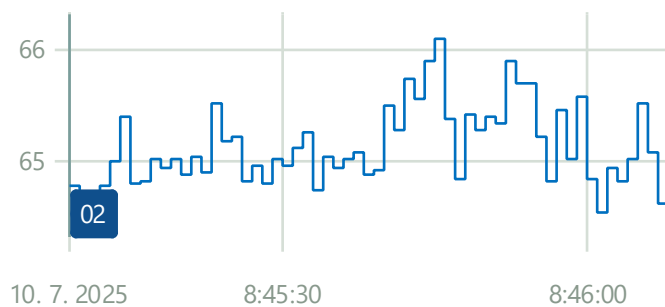
GRAF 10 Zobrazenie časového priebehu ekvivalentných hladín L_{Aeq,T} v meracom bode M10 – meranie čerpadla
