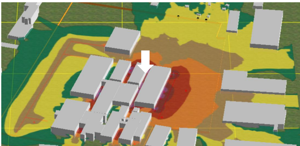
OBR. 13 3D model urbanistickej situácie v horizontálnom gride – bielou šípkou je zobrazený areál prevádzky COOPBOX Eastern, s.r.o. v Novom Meste nad Váhom
