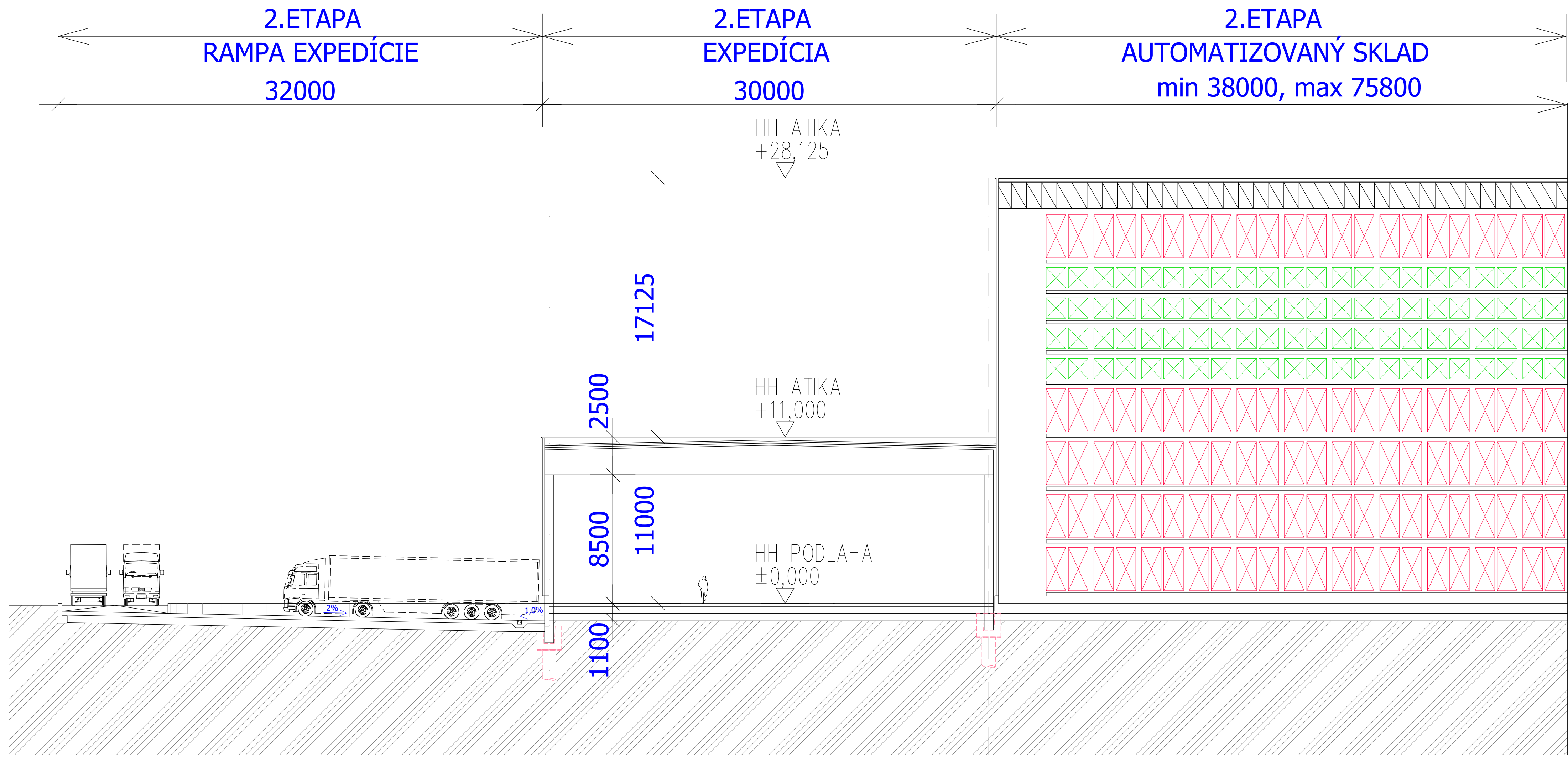
REZ C-C
