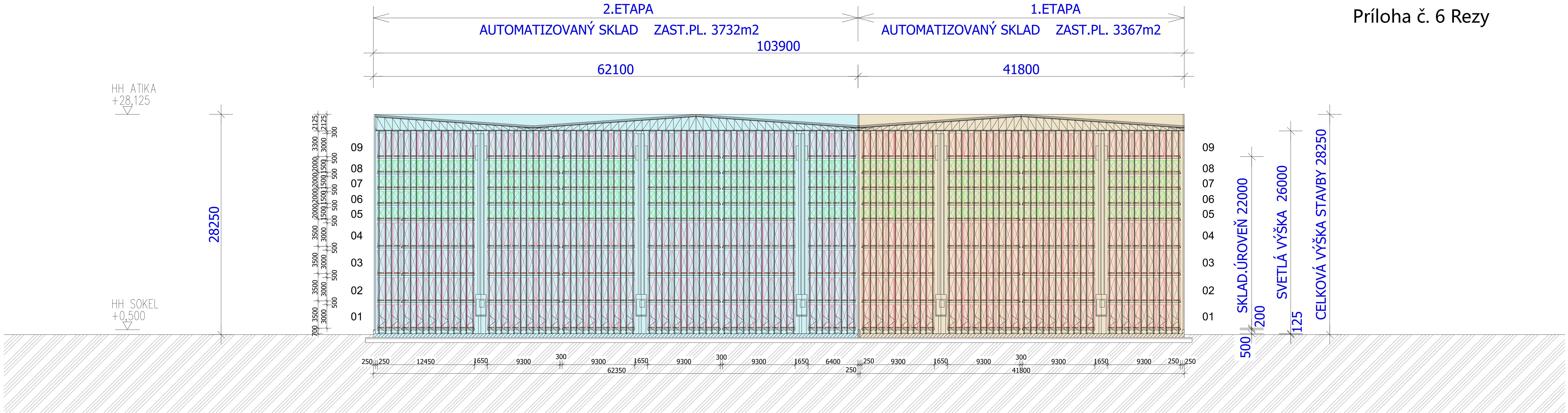
REZ A-A
