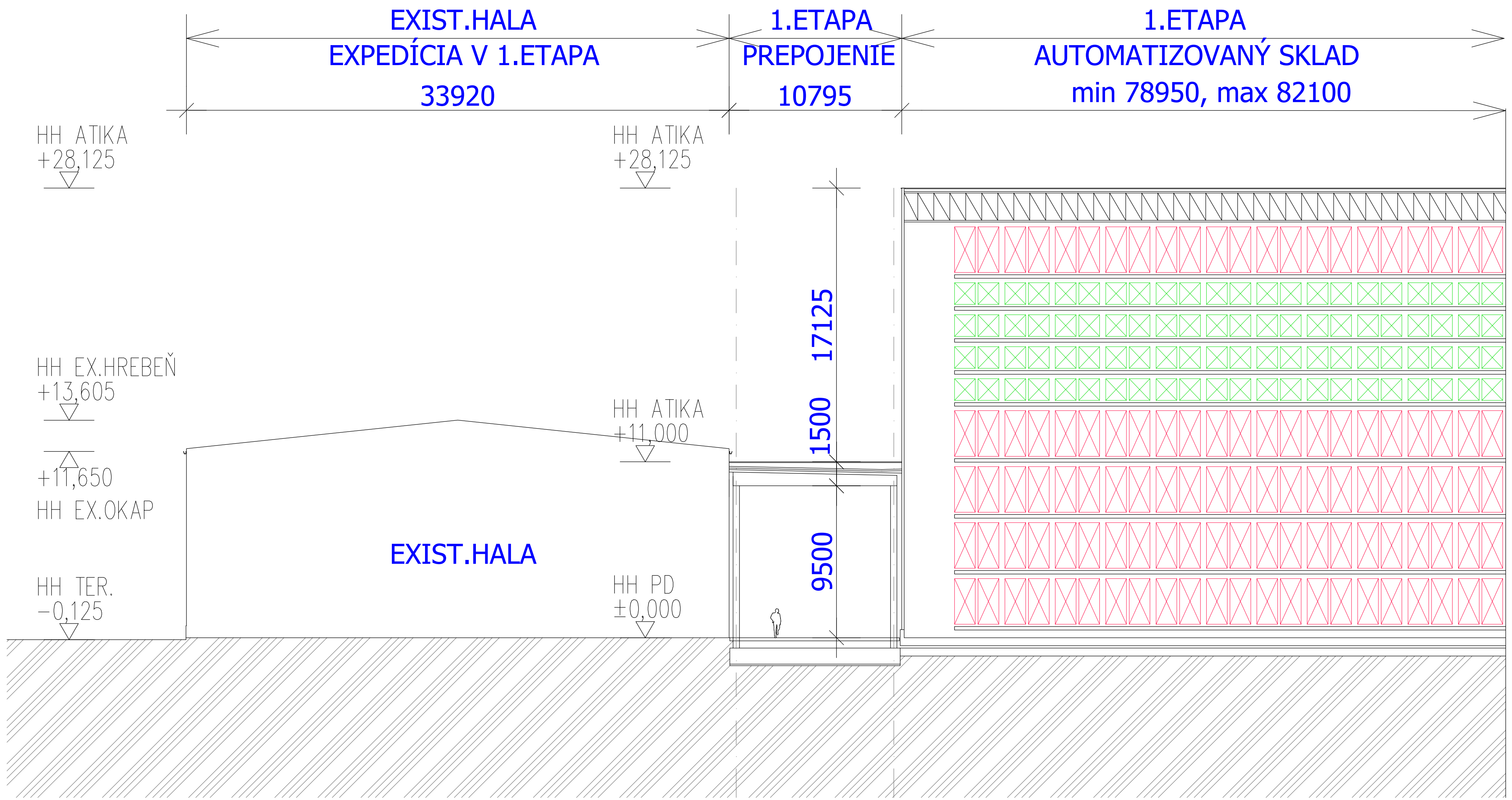
REZ B-B
