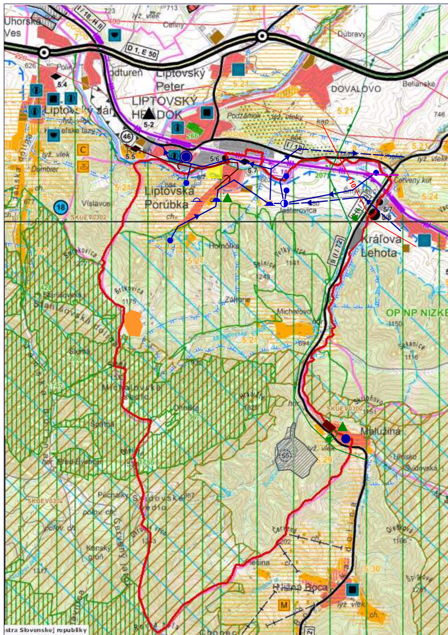
NÁVRH TECHNICKEJ INFRAŠTRUKTÚRY - ENERGETIKA
