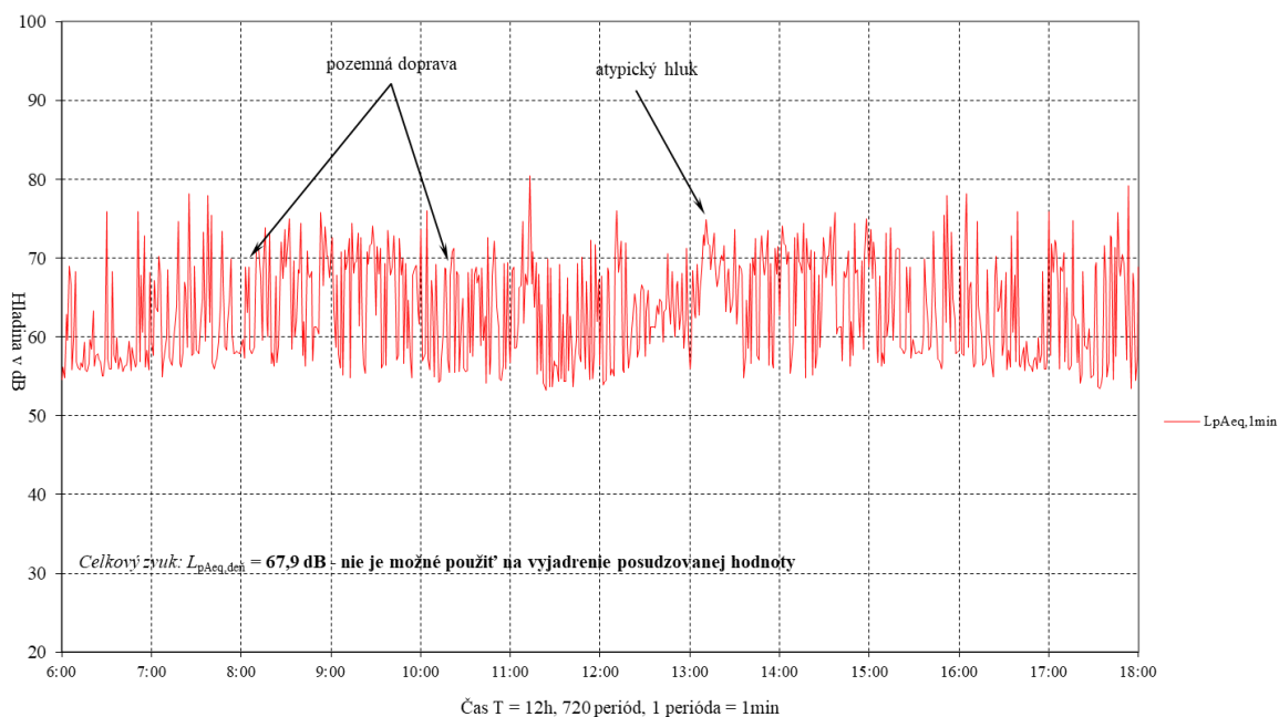
Obr. 4.3 Časový priebeh ekvivalentných hladín hluku L_{pAeq,1min} v referenčnom časovom intervale deň v čase T = 12h od 06:00 do 18:00 hod. dňa 28.01.2026 v meracom bode M1 .
