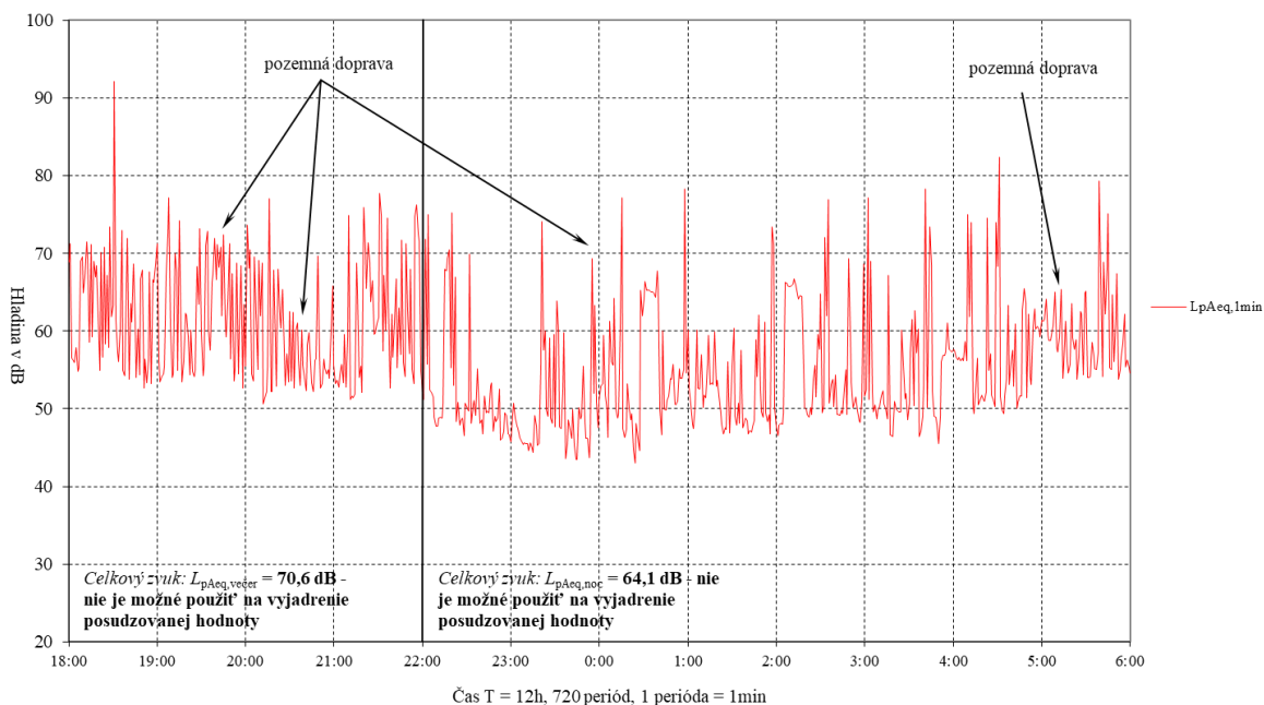
Obr. 4.4 Časový priebeh ekvivalentných hladín hluku L_{pAeq,1min} v referenčnom časovom intervale večer, v čase T = 4h od 18:00 hod do 22:00 hod dňa 27.01.2026 a v referenčnom časovom intervale noc, v čase T = 8h od 22:00 hod dňa 27.01.2026 do 06:00 hod dňa 28.01.2026 v meracom bode M1 .
