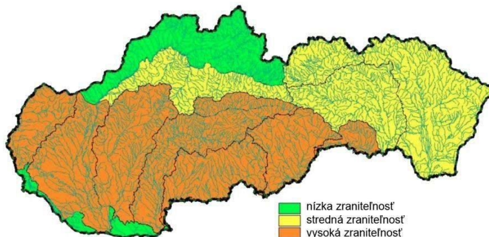
Obr. 2: Zraniteľnosť priemernej vodnosti Slovenska
