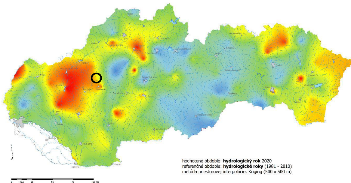
Obr. 3: Vývoj hydrologického roka z pohľadu podzemných vôd za rok 2020, SHMÚ
