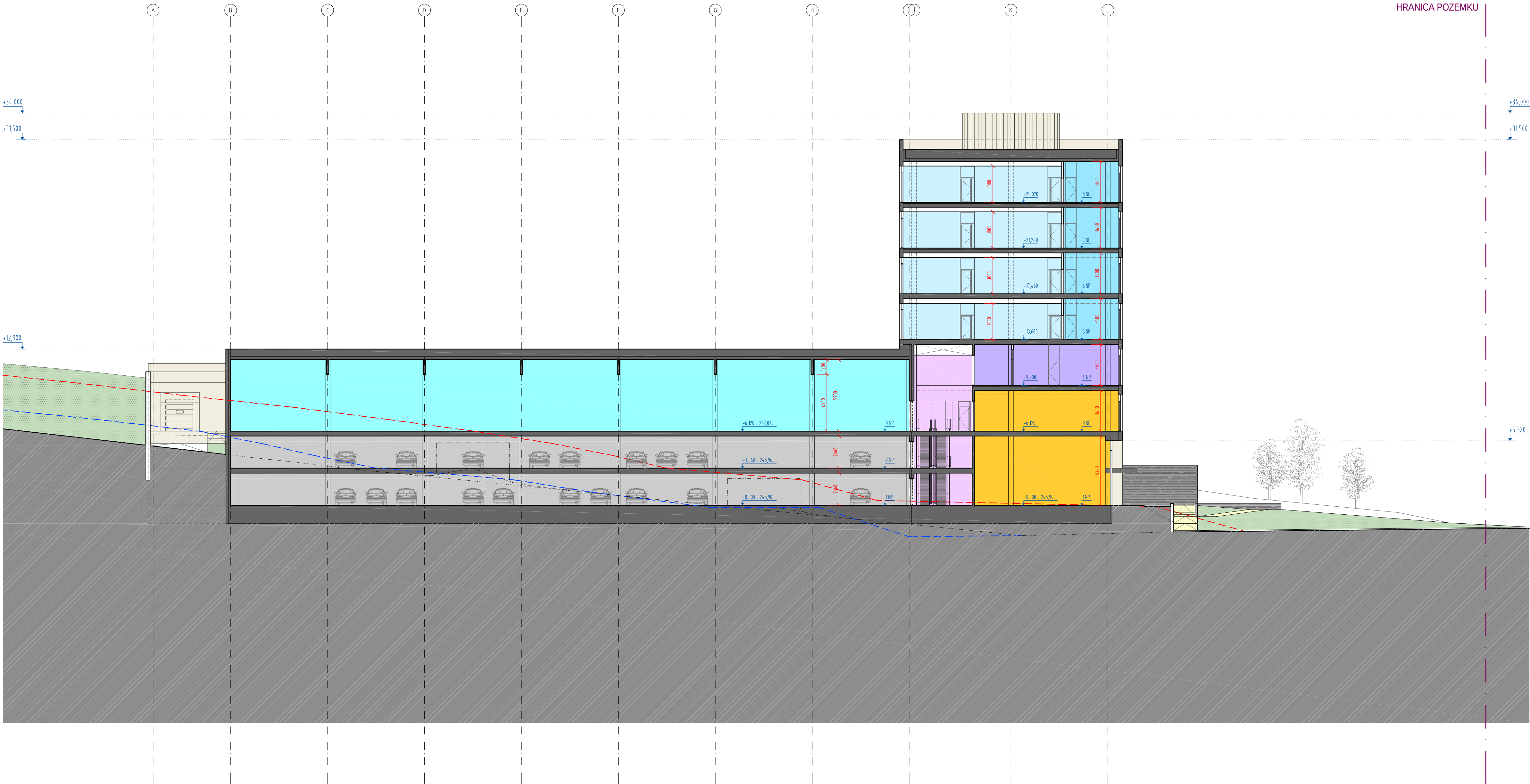
Príloha č.1a: Rez navrhovanou činnosťou - polyfunkčný objekt
