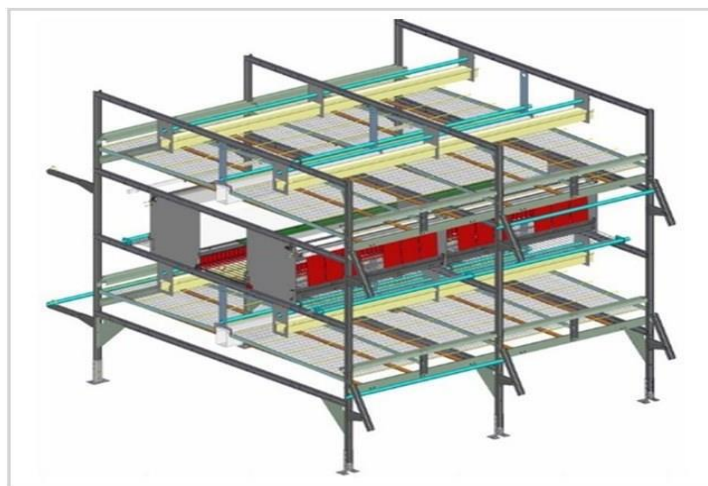
Obr.3 – voliérovy systém chovu pre haly č.4, č.5, č.6
