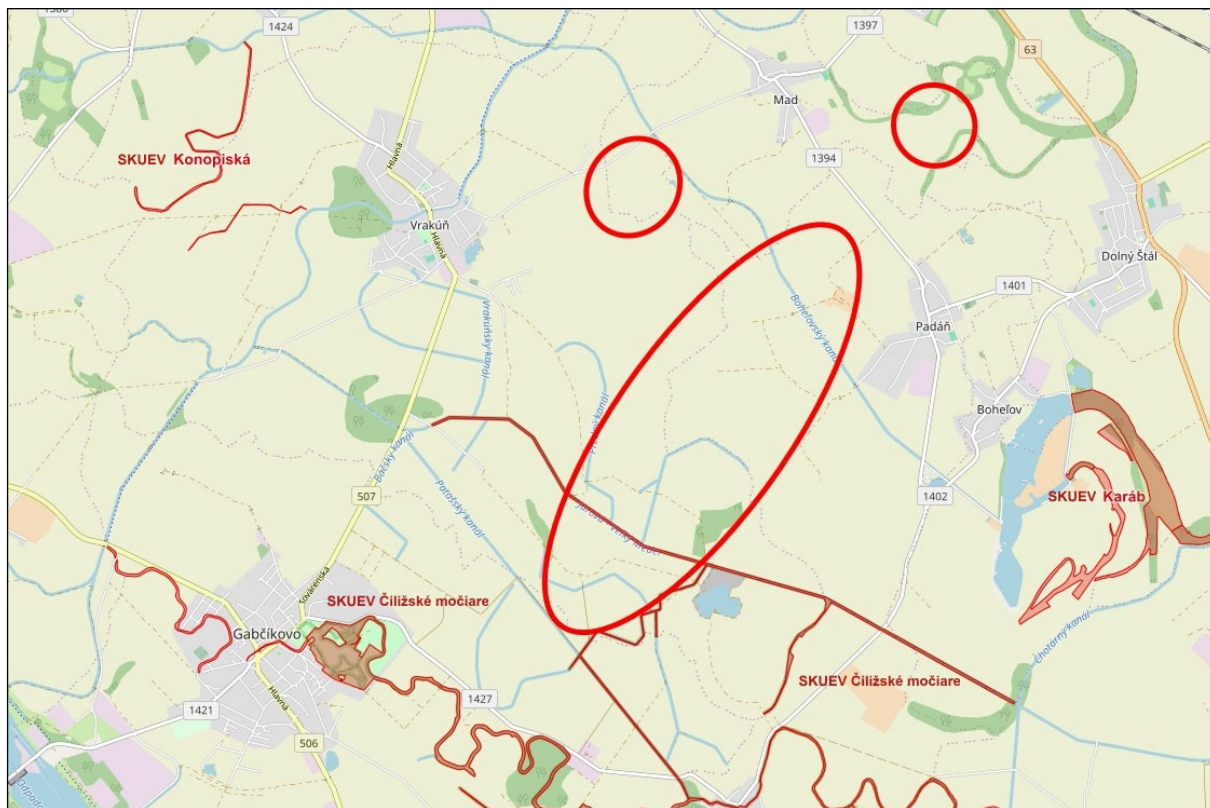
Obrázok 3: Umiestnenie navrhovanej činnosti vo vzťahu k chráneným územiám súvislej európskej sústavy chránených území NATURA 2000, lokalita umiestnenia VP vyznačená červenými elipsami.
