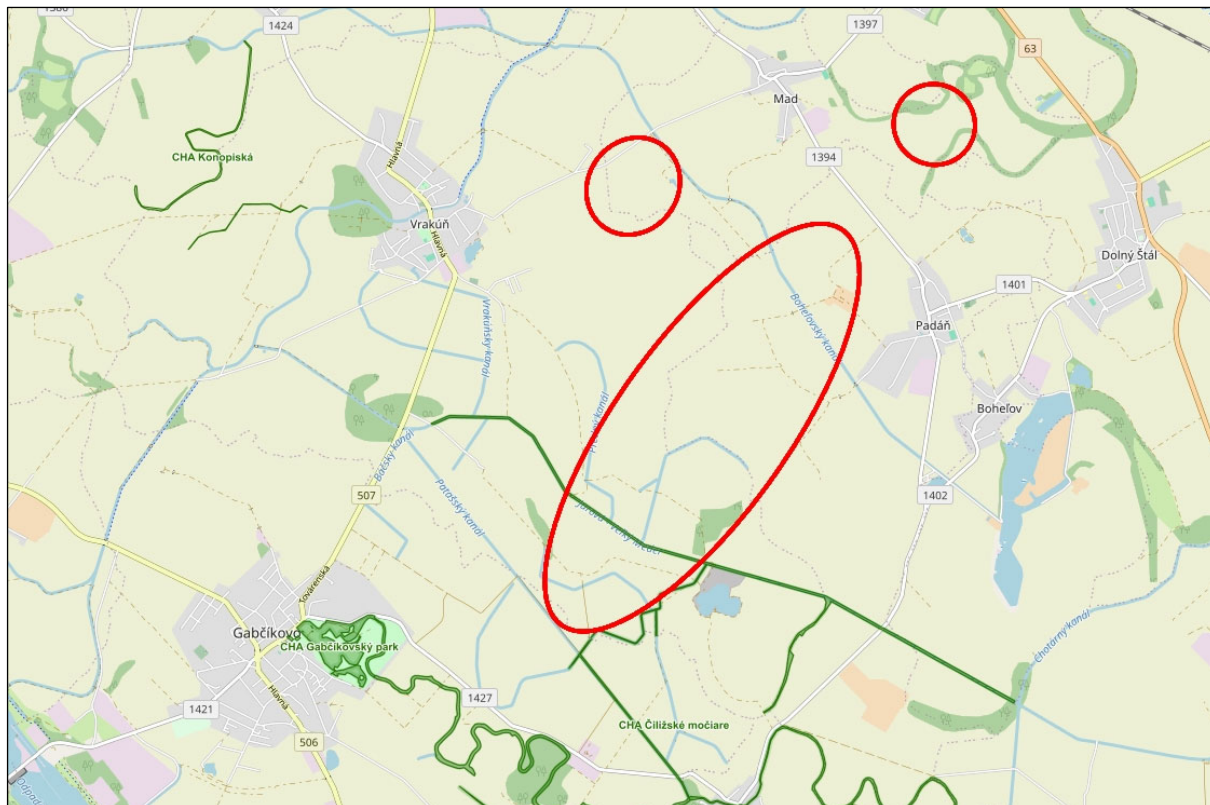
Obrázok 2: Umiestnenie navrhovanej činnosti vo vzťahu k chráneným územiám národnej siete chránených území, lokalita umiestnenia VP vyznačená červenými elipsami.
