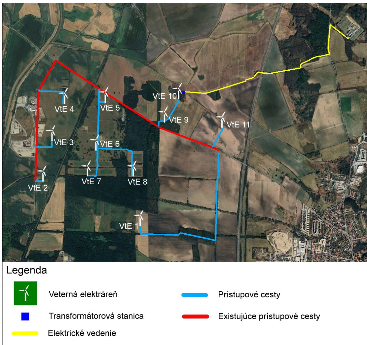
Obrázok 14: Trasovanie prístupových ciest a elektrického vedenia
