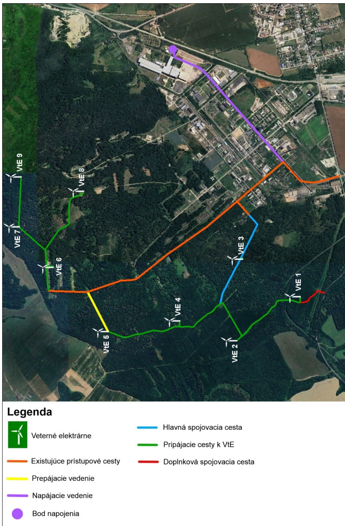
Obrázok 14: Trasovanie prístupových ciest a kabeláže
