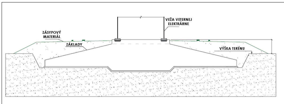
Obrázok 8: Teleso základov veternej elektrárne z armovaného betónu
