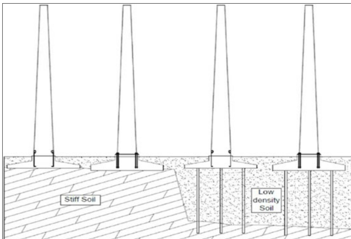
Obrázok 6: Spôsoby zakladania veterných elektrární v závislosti od finálneho geologického prieskumu
