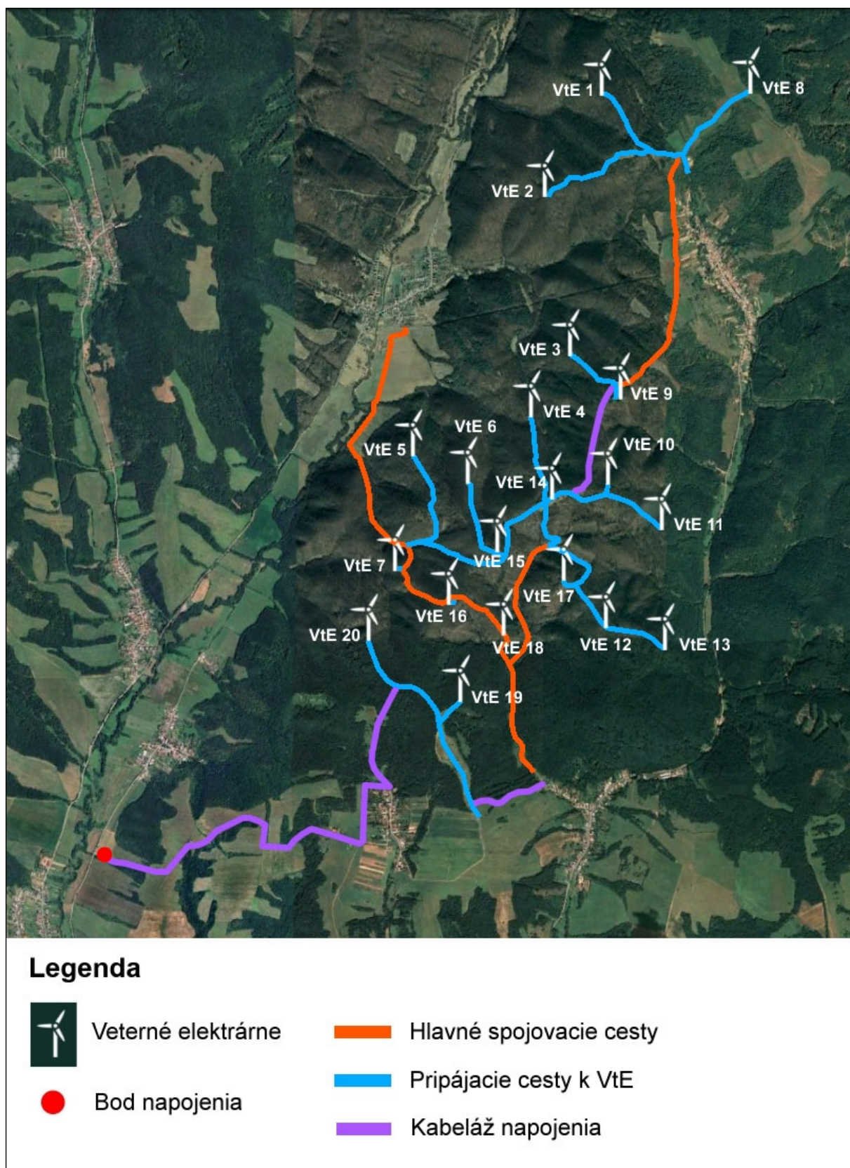
Obrázok 14: Trasovanie prístupových ciest a kabeláže
