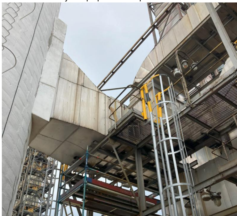
Obr.: Prvý vstup spalínového potrubia do komína
