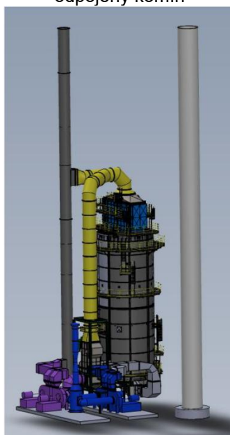
Obr.: Nový komín s výškou 60 m spolu so vzduchovo-spalinovým systémom napojeným na pec F1 a starý odpojený komín
