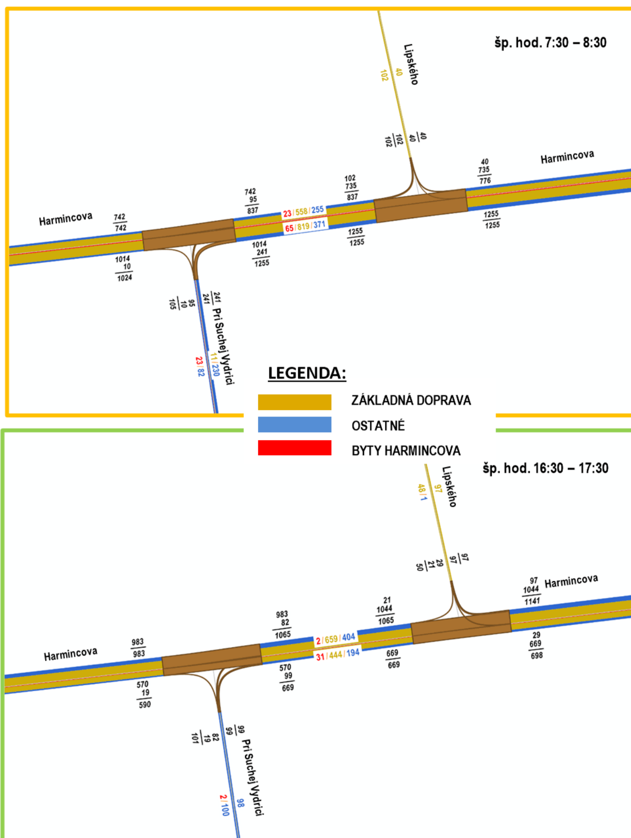
Obrázok č. 9: Zataženie križovatiek Harmincova – Pri Suchej Vydrici, Lipského
