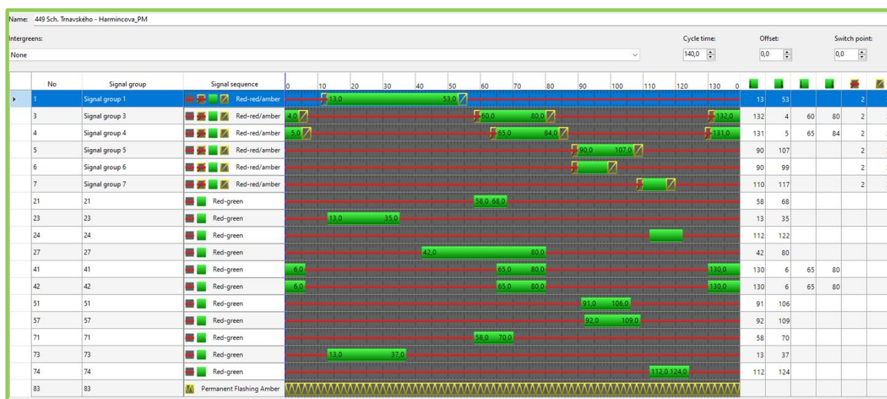
Obrázok č. 16: Signálny plán križovatky č. 449 Sch. Trnavského – Harmincova, popoludňajšia špička
