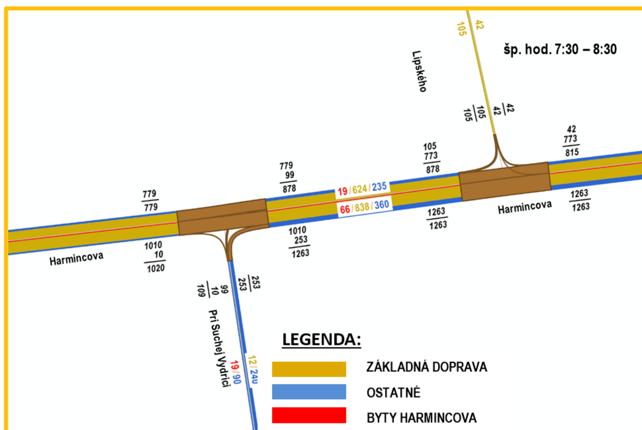
Obrázok č. 28: Zaťaženie križovatiek Harmincova – Pri Suchej Vydrici, Lipského, scenár 2045
