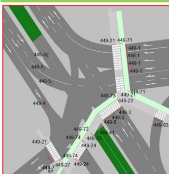
Obrázok č. 16: Signálny plán križovatky č. 449 Sch. Trnavského – Harmincova, popoludňajšia špička
