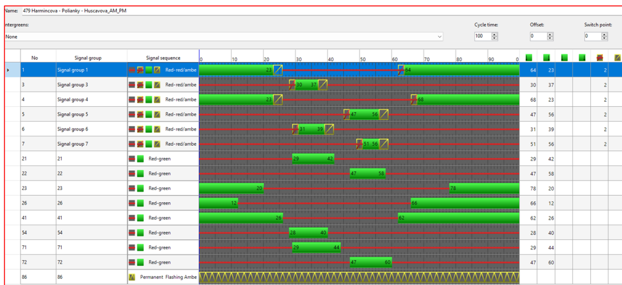
Obrázok č. 20: Signálny plán križovatky č. 479 Harmincova – Polianky, celodenný
