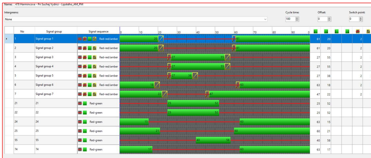
Obrazok č. 18: Signálny plán križovatky č. 478 Harmincova – Pri Suchej Vydrici - Lipského, celodenný
