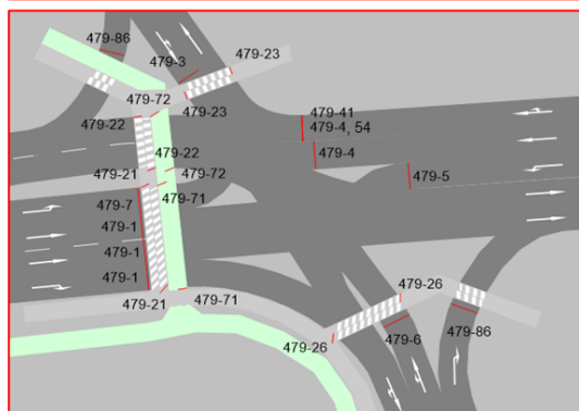
Obrázok č. 20: Signálny plán križovatky č. 479 Harmincova – Polianky, celodenný
