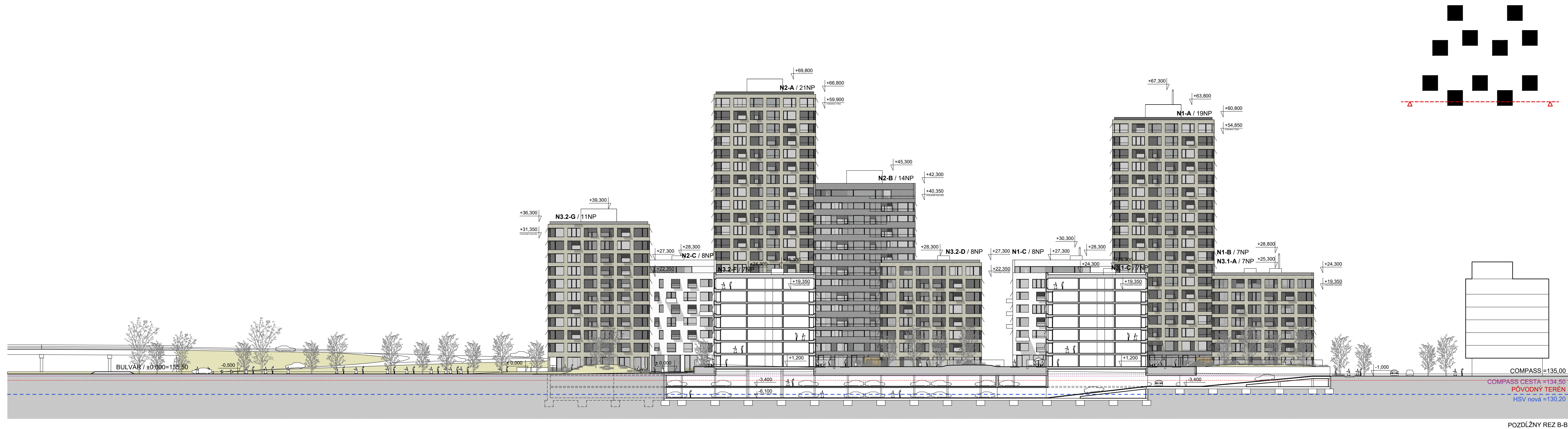
POZDĽŽNY REZ B-B
