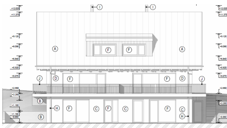
JUHOOZÁPADNÝ POHĽAD
