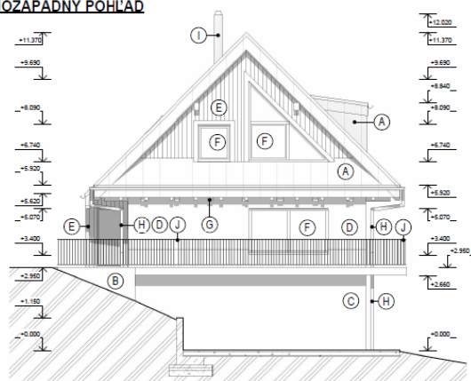
SEVEROZÁPADNÝ POHĽAD
