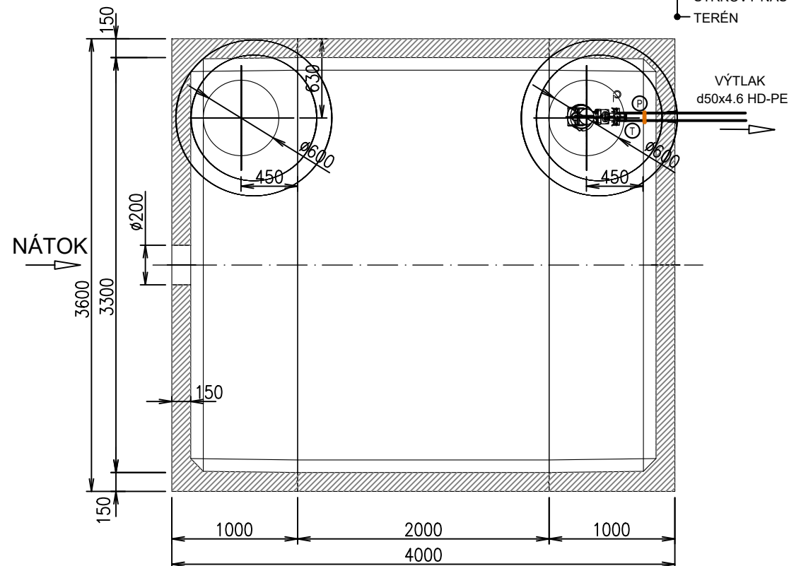
PÔDORYS
