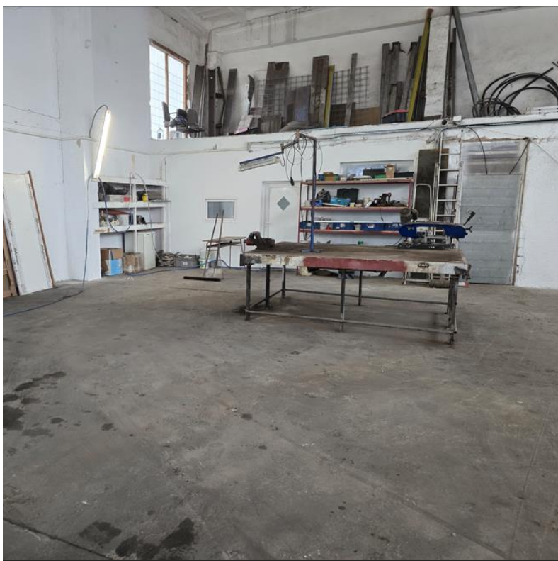
Obr.č.2 – pohľad na miesto ručného rozoberania elektroodpadov kategórie „O“ – 160214 a 200136 – pracovný stôl a ručné drobné náradie a elektrické náradie na demontáž
