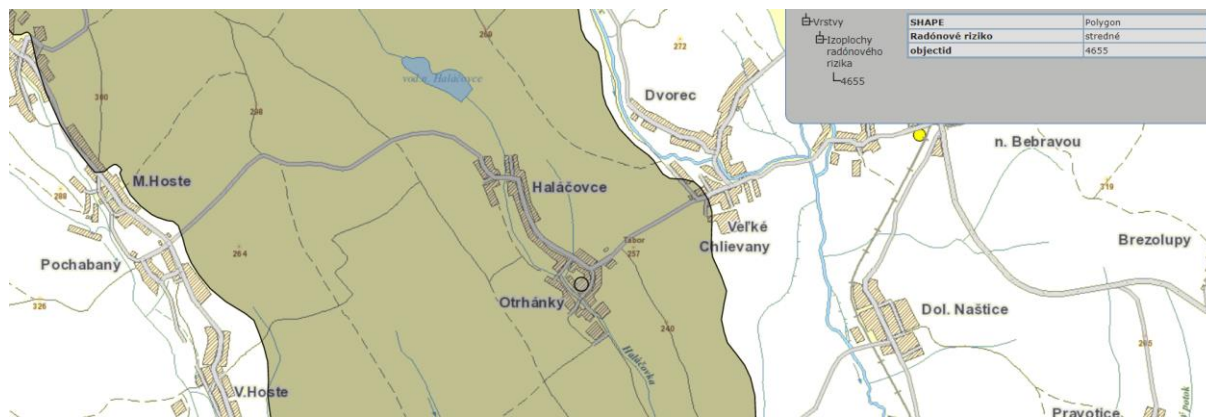
Obrázok: radónové riziko v obci Otrhánky Zdroj: 20.5.2025, https://apl.geology.sk/radio/
