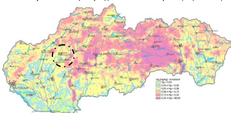
Obrázok: Výskyt Ortuti v pôde - A horizont v regióne Zdroj: http://apl.geology.sk/atlaspydy/
