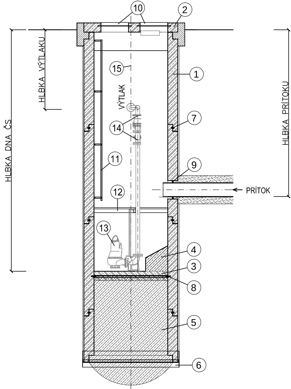
ČERPACIA STANICA - REZ A-A M 1:50
