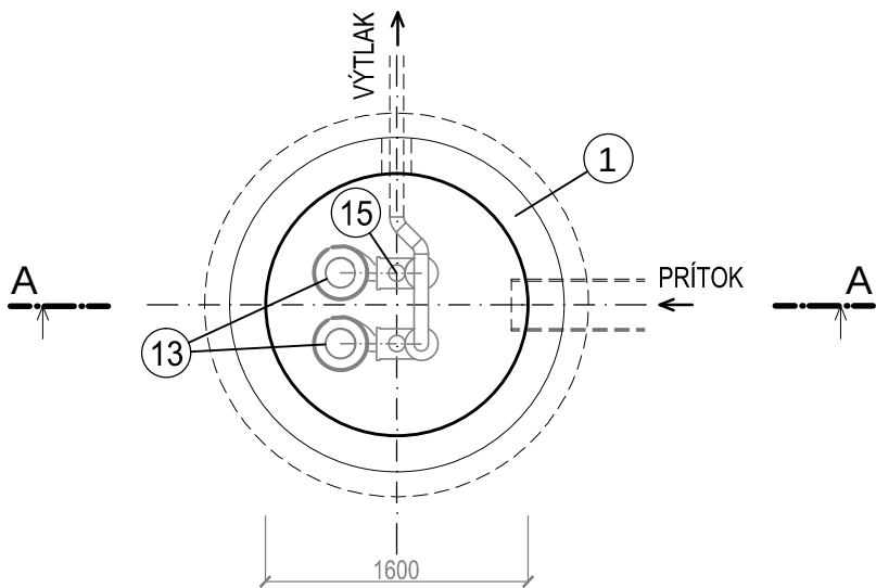
ČERPACIA STANICA - PÔDORYSNÝ REZ M 1:50
