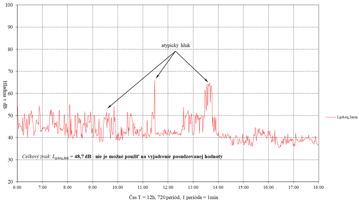
Obr. 4.3 Časový priebeh ekvivalentných hladín hluku L_{pAeq,1min} v referenčnom časovom intervale deň v čase T = 12h od 06:00 do 18:00 hod. dňa 29.04.2025 v meracom bode M1 .
