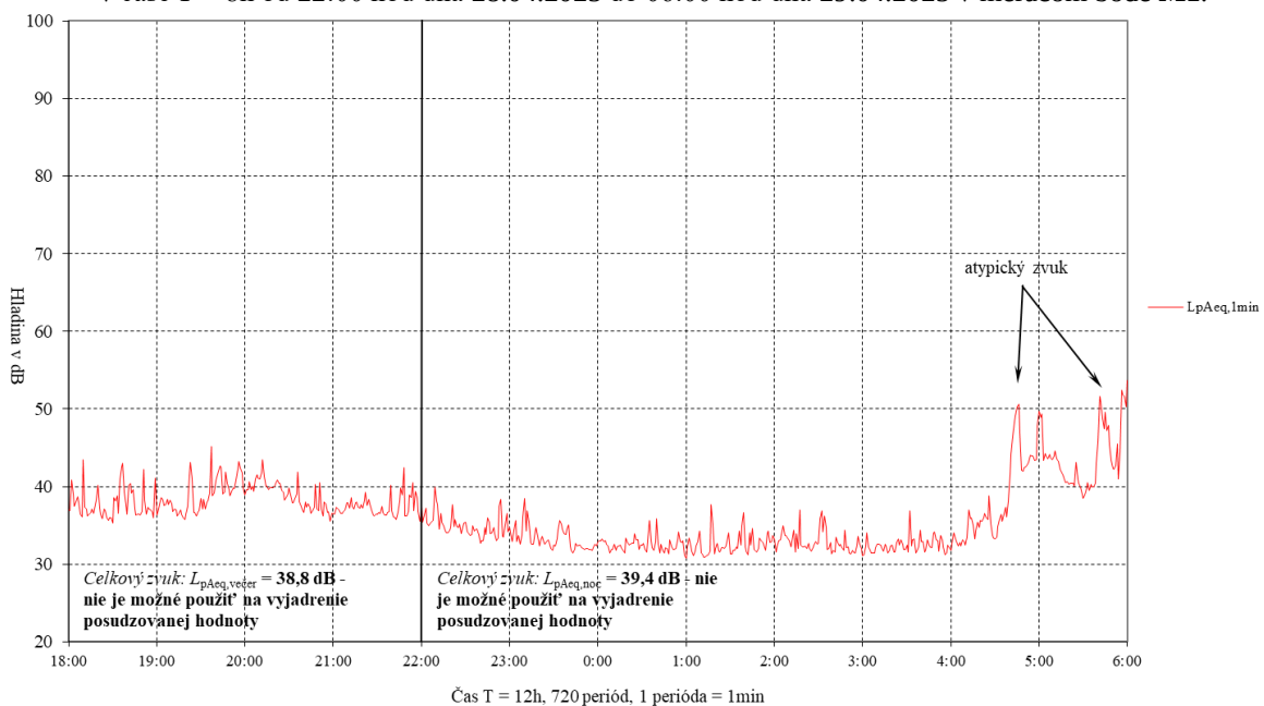
Obr. 4.4 Časový priebeh ekvivalentných hladín hluku L_{pAeq,1min} v referenčnom časovom intervale večer, v čase T = 4h od 18:00 hod do 22:00 hod dňa 28.04.2025 a v referenčnom časovom intervale noc, v čase T = 8h od 22:00 hod dňa 28.04.2025 do 06:00 hod dňa 29.04.2025 v meracom bode M1 .
