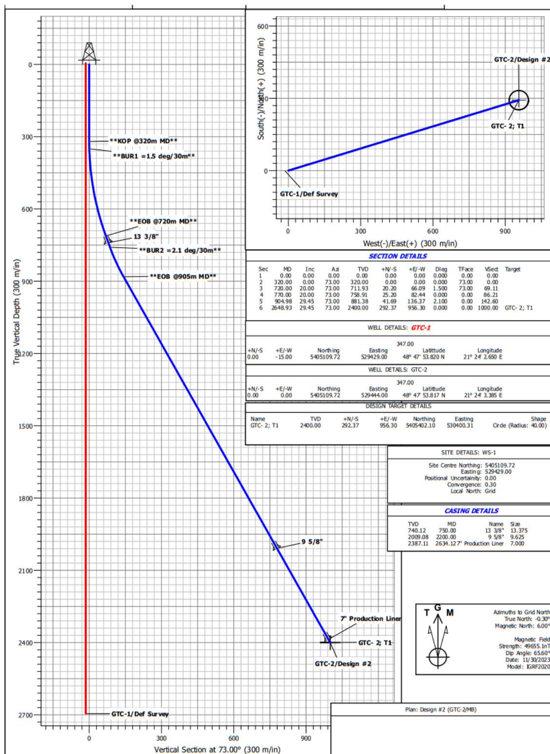
Obr. 9 Technický profil plánovaného vrtu
