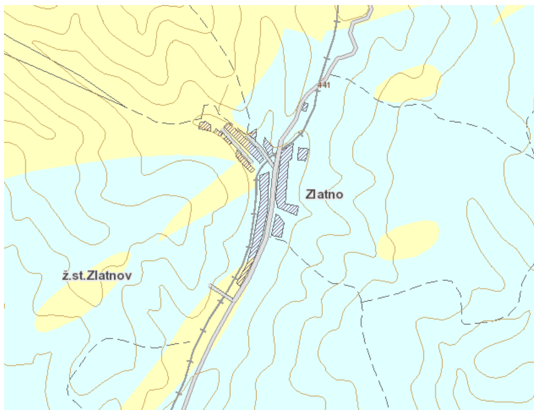
Obrázok 6: Mapa prírodnej rádioaktivity
