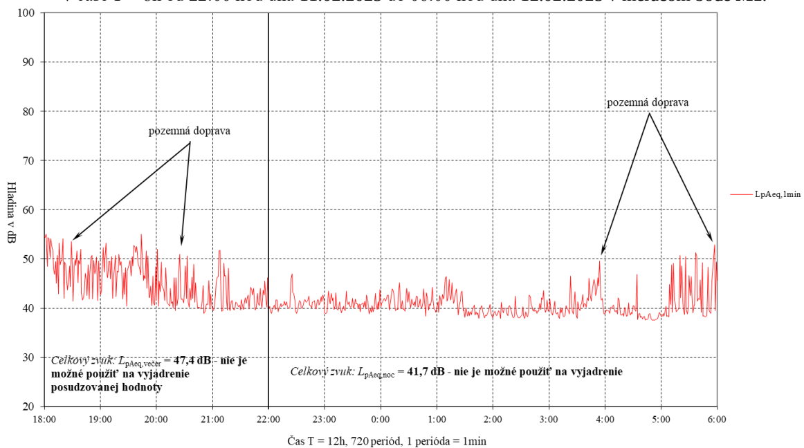
Obr. 4.4 Časový priebeh ekvivalentných hladín hluku L_{pAeq,1min} v referenčnom časovom intervale večer, v čase T = 4h od 18:00 hod do 22:00 hod dňa 11.02.2025 a v referenčnom časovom intervale noc, v čase T = 8h od 22:00 hod dňa 11.02.2025 do 06:00 hod dňa 12.02.2025 v meracom bode M1 .
