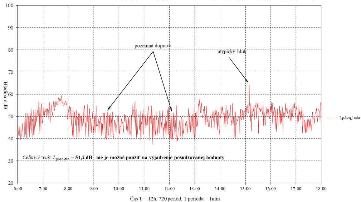
Obr. 4.3 Časový priebeh ekvivalentných hladín hluku L_{pAeq,1min} v referenčnom časovom intervale deň v čase T = 12h od 06:00 do 18:00 hod. dňa 11.02.2025 v meracom bode M1 .
