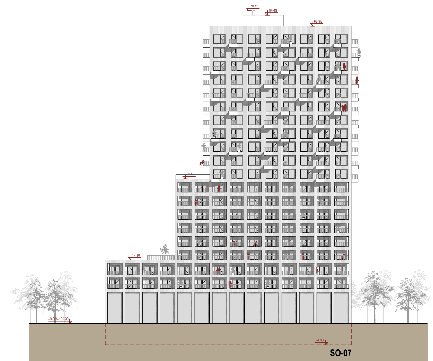
BOČNÉ POHL'ADY - SO-07
