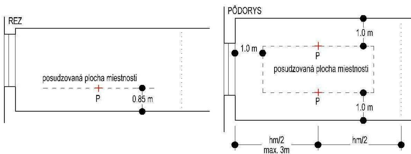
Rozloženie kontrolných bodov vo vnútornom priestore na horizontálnej zrovnávacej rovine.
