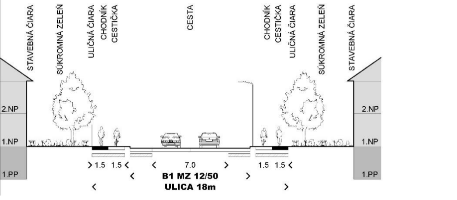
obr. 95 Profil priestranstva, ktorý slúži ako tranzit a súčasne ako prístup k zástavbe (PFČasti 402, 403, 404, 405, 503, 504, 702, 801.).
