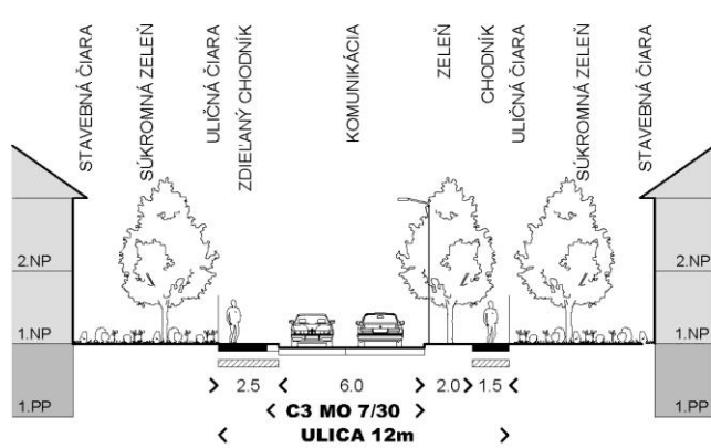
obr. 107 Profil priestranstva, ktorý slúži ako prístup k zástavbe, obytná ulica.
