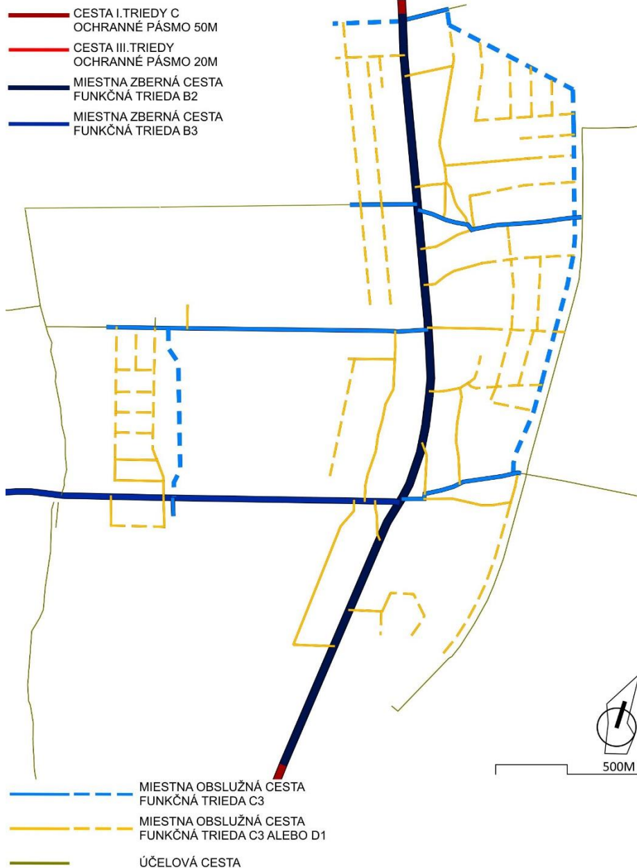
obr. 113 Miestny komunikačný systém (hlavné územie obce) Variant 1
