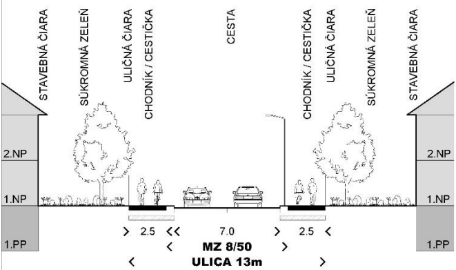
obr. 98 Profil priestranstva, ktorý slúži ako tranzit a súčasne ako prístup k zástavbe (PFČasti 403, 602, 603, 901 (Staničná ulica)).
