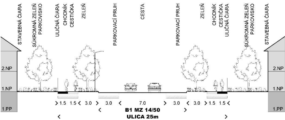
obr. 96 Profil priestranstva, ktorý slúži ako tranzit a súčasne ako prístup k zástavbe (PFČasti Seget a Arkuš (801, 702).
