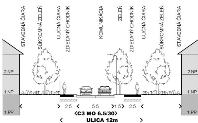
obr. 99 Profil priestranstva, ktorý je súčasťou významných obecných koridorov.
