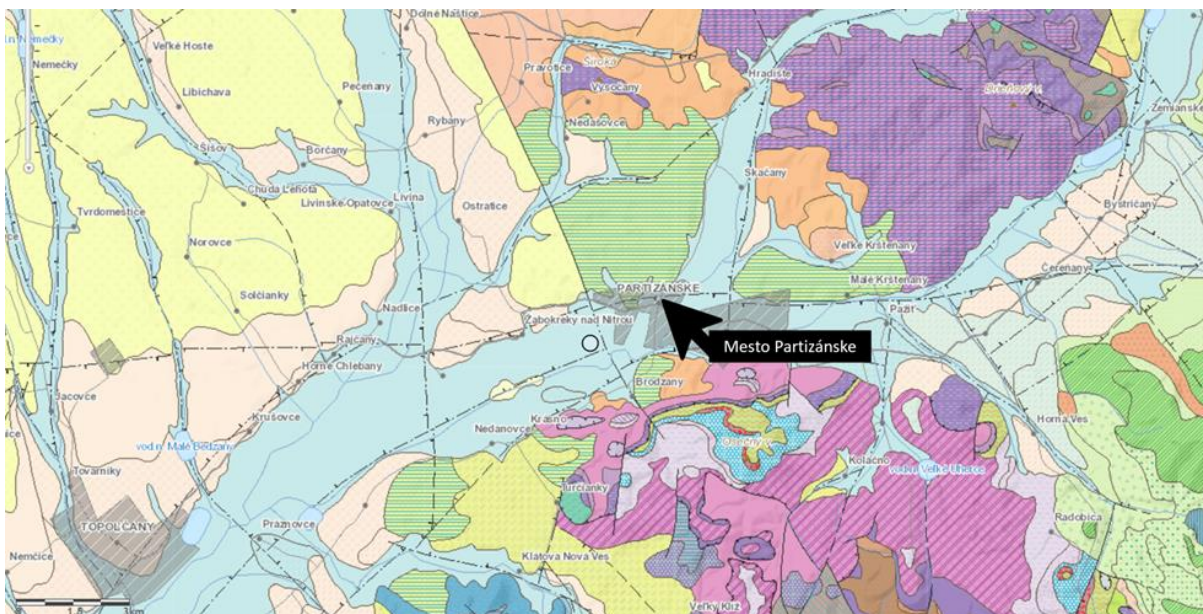
Obrázok 14 Prehľad geologického podložia mesta Partizánske
