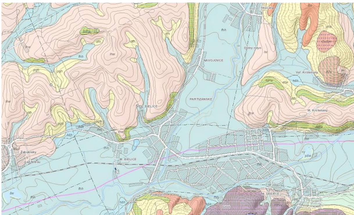
Obrázok 13 Geologická mapa územia mesta Partizánske a jeho okolie
