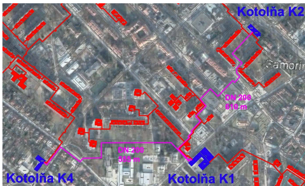
Obrázok 9 Plánované prepojenie tepelných okruhov v CZT
