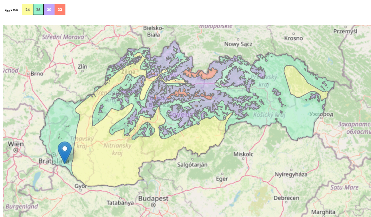
Obrázok 6 Výskyt veternej energie na Slovensku, mesto Šamorín
