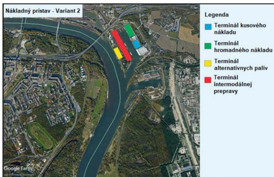
Obrázok 2: Variant 2 – koncentrácia prekládkových aktivít v Pálenisku
