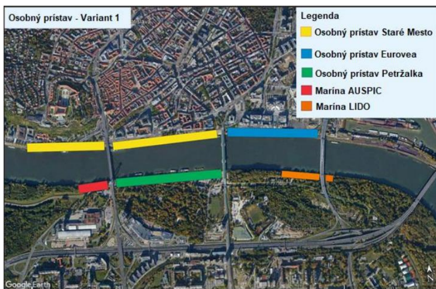
Obrázok 4: Variant 1 – voľný tok na Dunaji
