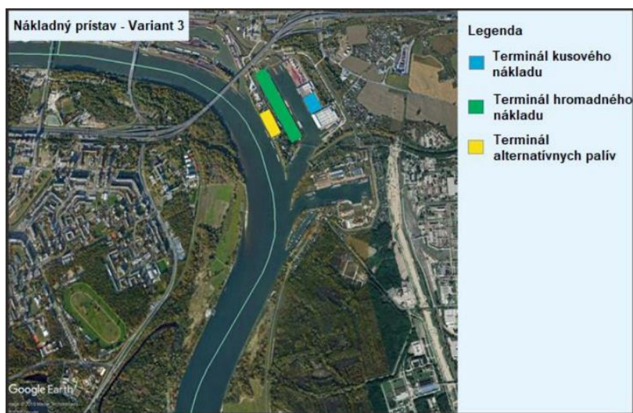
Obrázok 3: Variant 3 – koncentrácia prekládkových aktivít v Pálenisku
