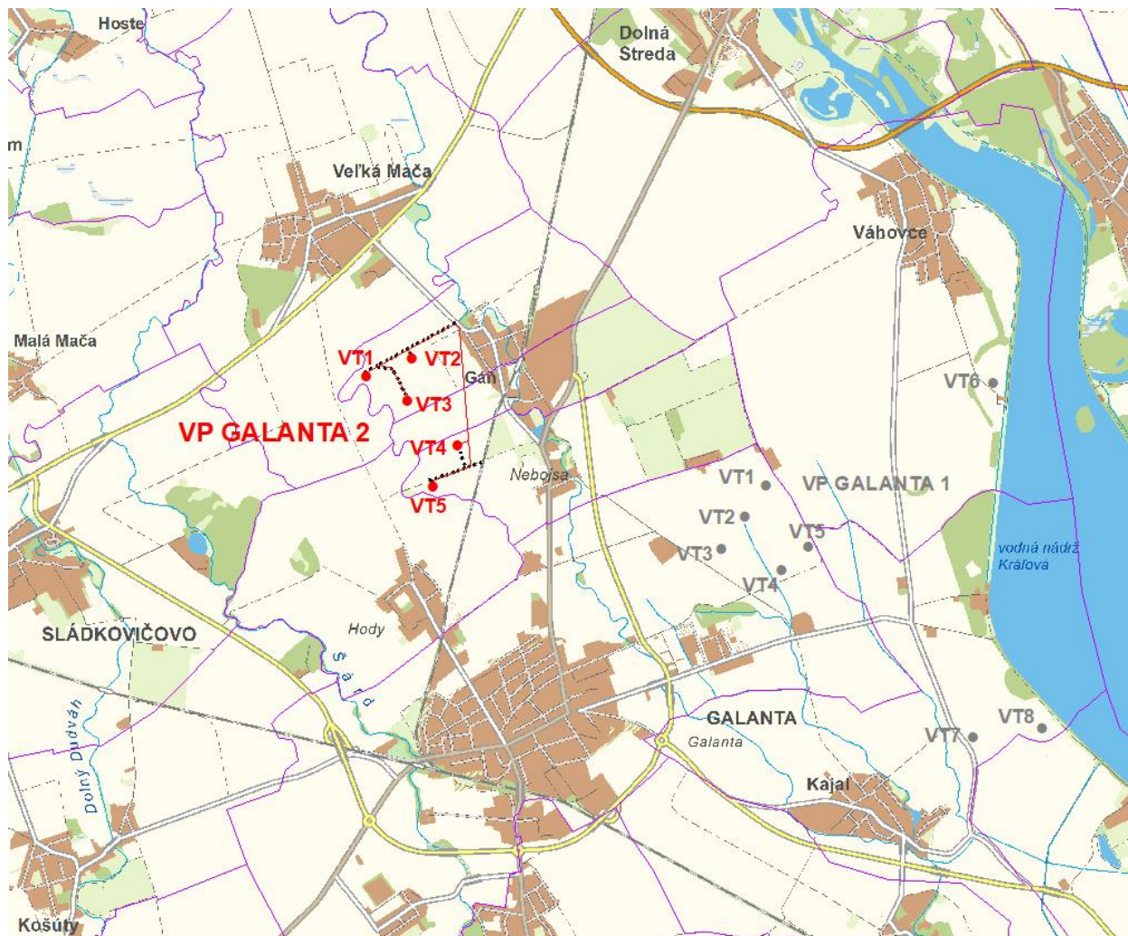
Obr. 1 Lokalizácia navrhovaného veterného parku Galanta 2
