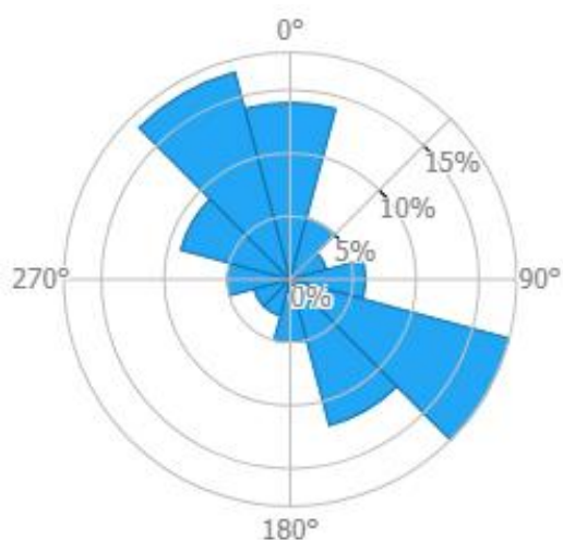
Obr. 4 Relatívna početnosť výskytu smerov vetra v riešenom území
