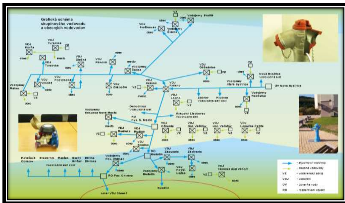
Obrázok 16: Grafická schéma skupinového vodovodu a obecných vodovodov
