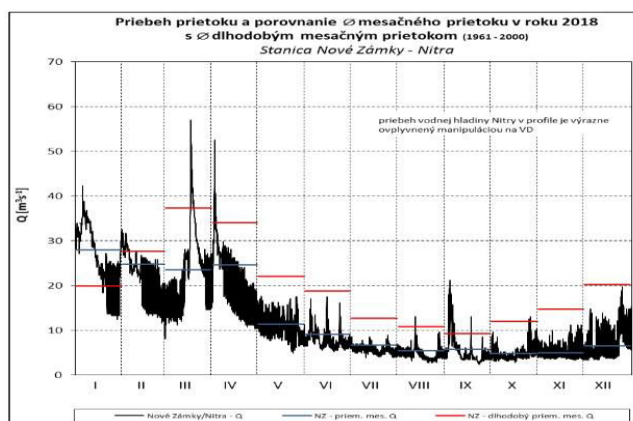
Obr.3 Priebeg prietoku na stanici Nové Zámky – Nitra v roku 2018 (Zdroj: SHMU).
