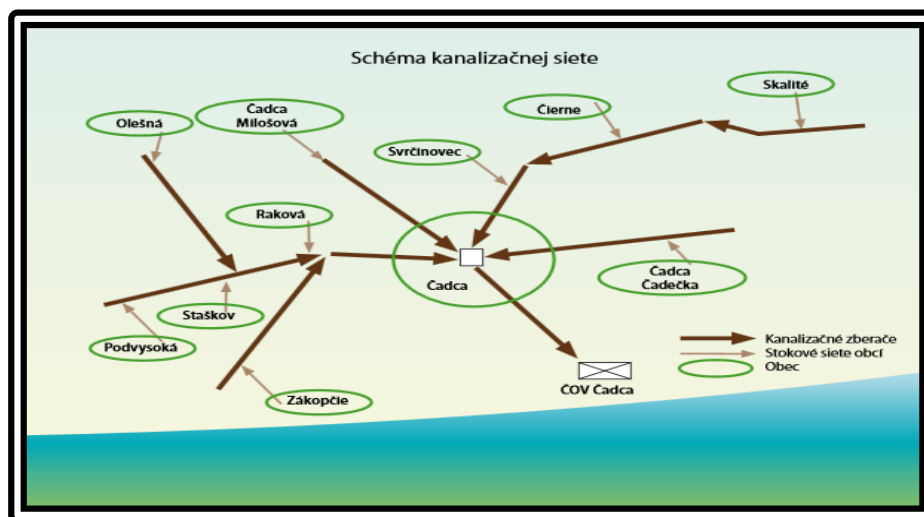
Obrázok 17: Schéma skupinovej kanalizačnej siete Čadca - ČOV Čadca
