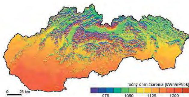
Obr.12: Slniečny svit na území Slovenska.
