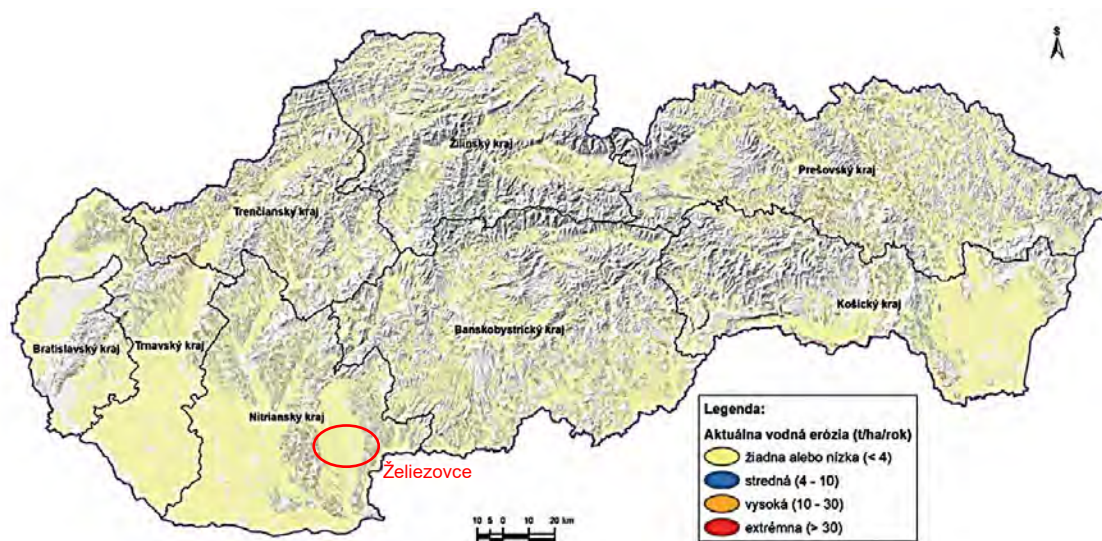
Obr. 30: Aktuálna vodná erózia na poľnohospodárskej pôde (2021)
