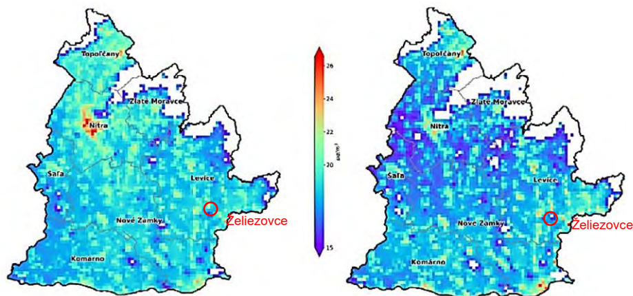
Obr.24: Priemerná ročná koncentrácia PM10 (vľavo) a počet prekročení limitnej dennej hodnoty PM10 (vpravo) v roku 2021. Zobrazené sú len hodnoty nad 15 \mu\text{g}\cdot\text{m}^{-3} a nenulový počet prekročení.
