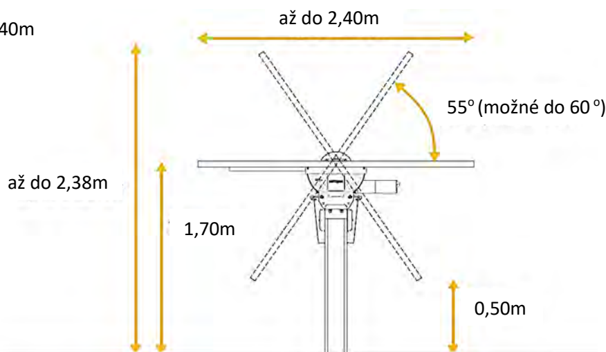
Obr. 8: Nezávislý horizontálny sledovač s jednou osou
