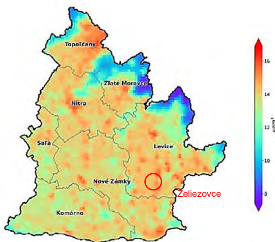
Obr.25: Priemerné ročné koncentrácie PM2,5 v roku 2021. Zobrazené sú len hodnoty vyššie ako 5 \mu\text{g}\cdot\text{m}^{-3} , čo je limitná hodnota odporúčaná WHO.
