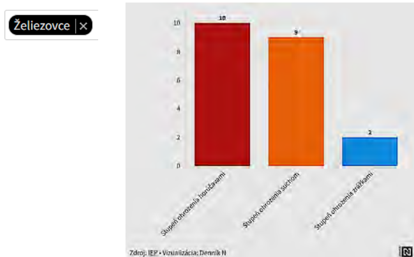
Graf 1 : Stupeň ohrozenia prírodnými vplyvmi v oblasti Želiezoviec
