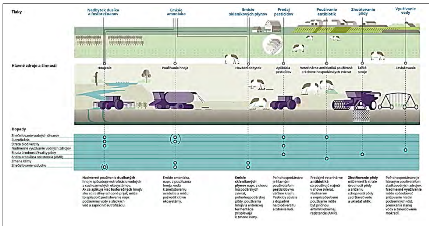
Obr. 29: Poľnohospodárstvo – Cyklus znečisťovania a ďalšie dopady na životné prostredie
