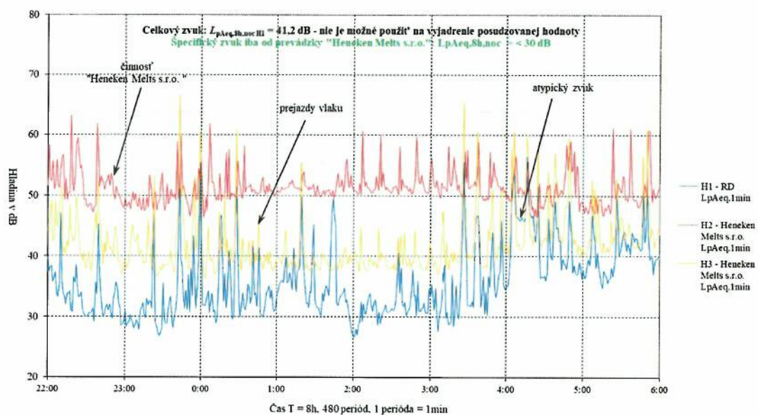
Obr. 4.2 Časový priebeh ekvivalentných hladín hluku L_{pAeq,1min} v meracích bodoch H1, H2 a H3 pre referenčný časový interval noc (od 22:00 hod. do 06:00 hod.) 24.-25.05.2022.
