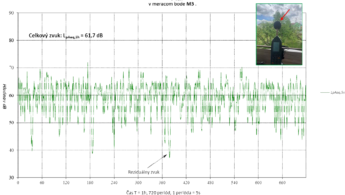
Obr. 3.13 Informatívny časový priebeh ekvivalentných hladín hluku L_{pAeq,5s} v čase T = 1 hod. od 09:00 hod do 10:00 hod. zo dňa 31.05.2025 v meracom bode M3.
