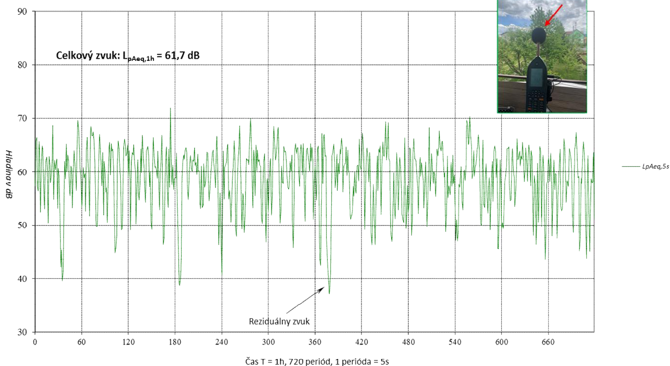
Obr. 3.13 Informatívny časový priebeh ekvivalentných hladín hluku L_{pAeq,5s} v čase T = 1 hod. od 09:00 hod do 10:00 hod. zo dňa 31.05.2025 v meracom bode M3.
