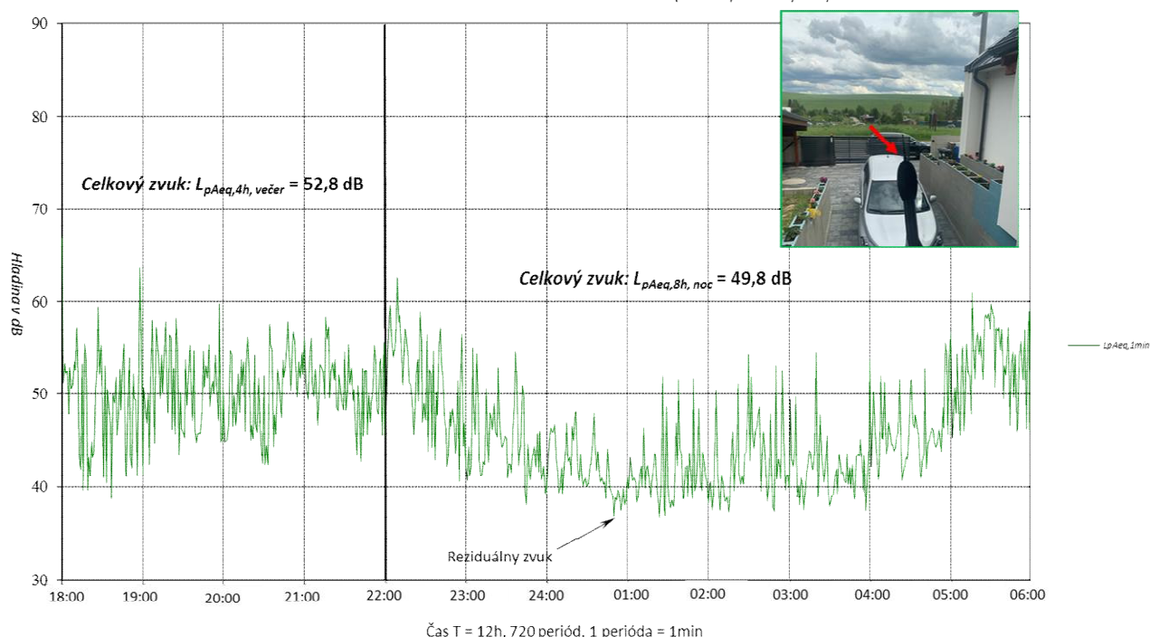
Obr. 3.4 Časový priebeh ekvivalentných hladín hluku L_{pAeq,1min} v čase T = 12 hod. od 18:00 hod dňa 30.05.2022 do 06:00 hod. dňa 31.05.2022 v meracom bode M1 . (večerný a nočný čas)
