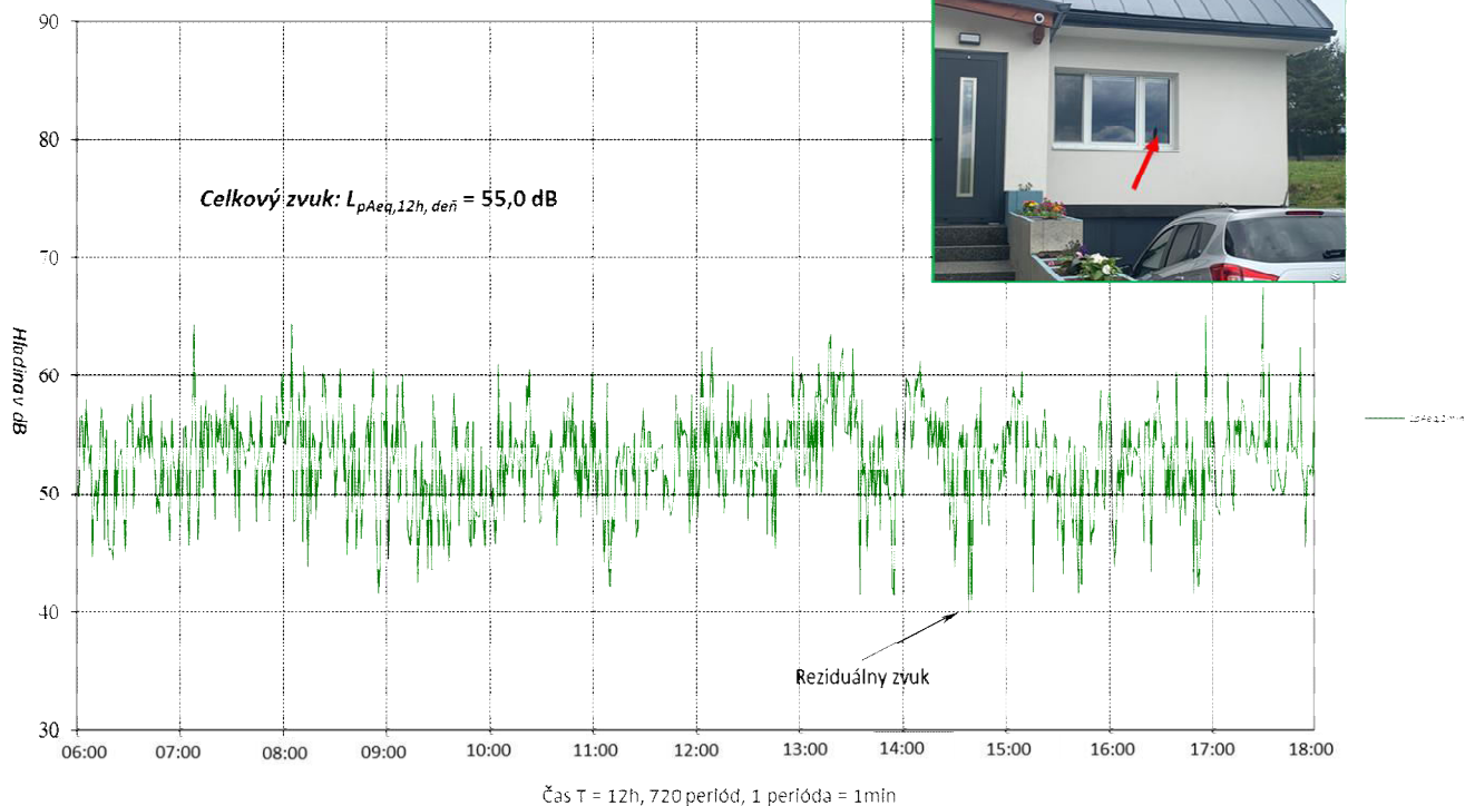
Obr. 3.5 Časový priebeh ekvivalentných hladín hluku L_{pAeq,1min} v čase T = 12 hod. od 06:00 hod do 18:00 hod. dňa 31.05.2022 v meracom bode M1. (denný čas)
