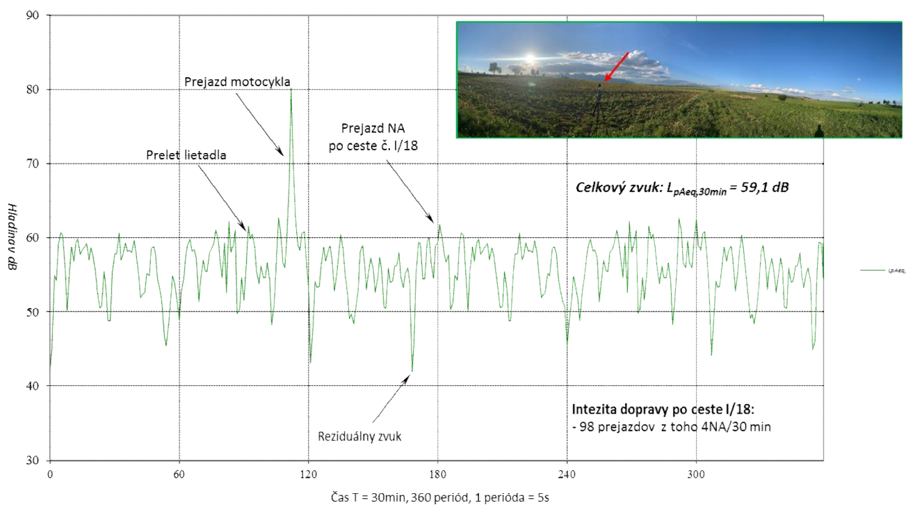
Obr. 3.14 Informatívny časový priebeh ekvivalentných hladín hluku L_{pAeq,5s} v čase T = 30 min. od 19:00 hod. do 19:30 hod. zo dňa 31.05.2022 v meracom bode M4.
