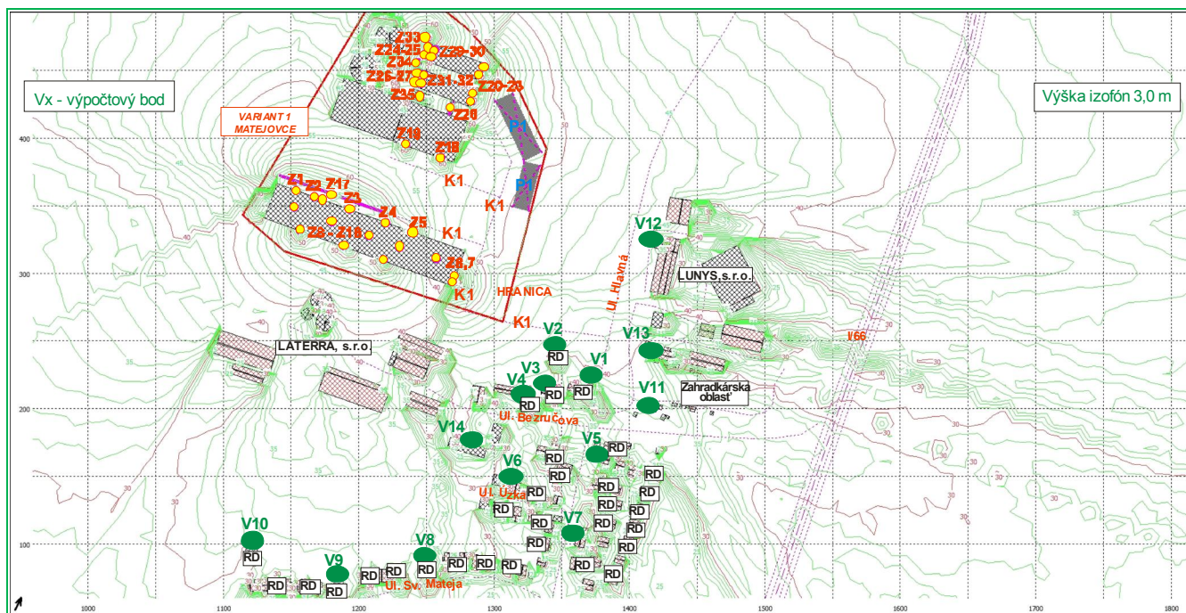
Obr. 2.5 Grafický výstup z programu HLUK + profi verzia 11 Hluková situácia záujmového územia pre noc - L_{pAeq,8h} v čase od 22:00 - 06:00 hod., situácia iba od činnosti projektu „CENTRUM ENERGETICKÉHO A BIOLOGICKÉHO ZODNOTENIA ODPADU - VARIANT 1 MATEJOVCE“, A – variant
