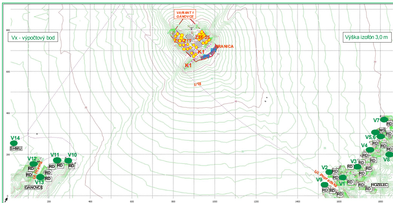
Obr. 2.5 Grafický výstup z programu HLUK + profi verzia 11 Hluková situácia záujmového územia pre deň - L_{pAeq,12h} v čase od 06:00 - 18:00 hod., situácia iba od činnosti projektu „CENTRUM ENERGETICKÉHO A BIOLOGICKÉHO ZODNOTENIA ODPADU - VARIANT 2 GÁNOVCE“, A – variant
