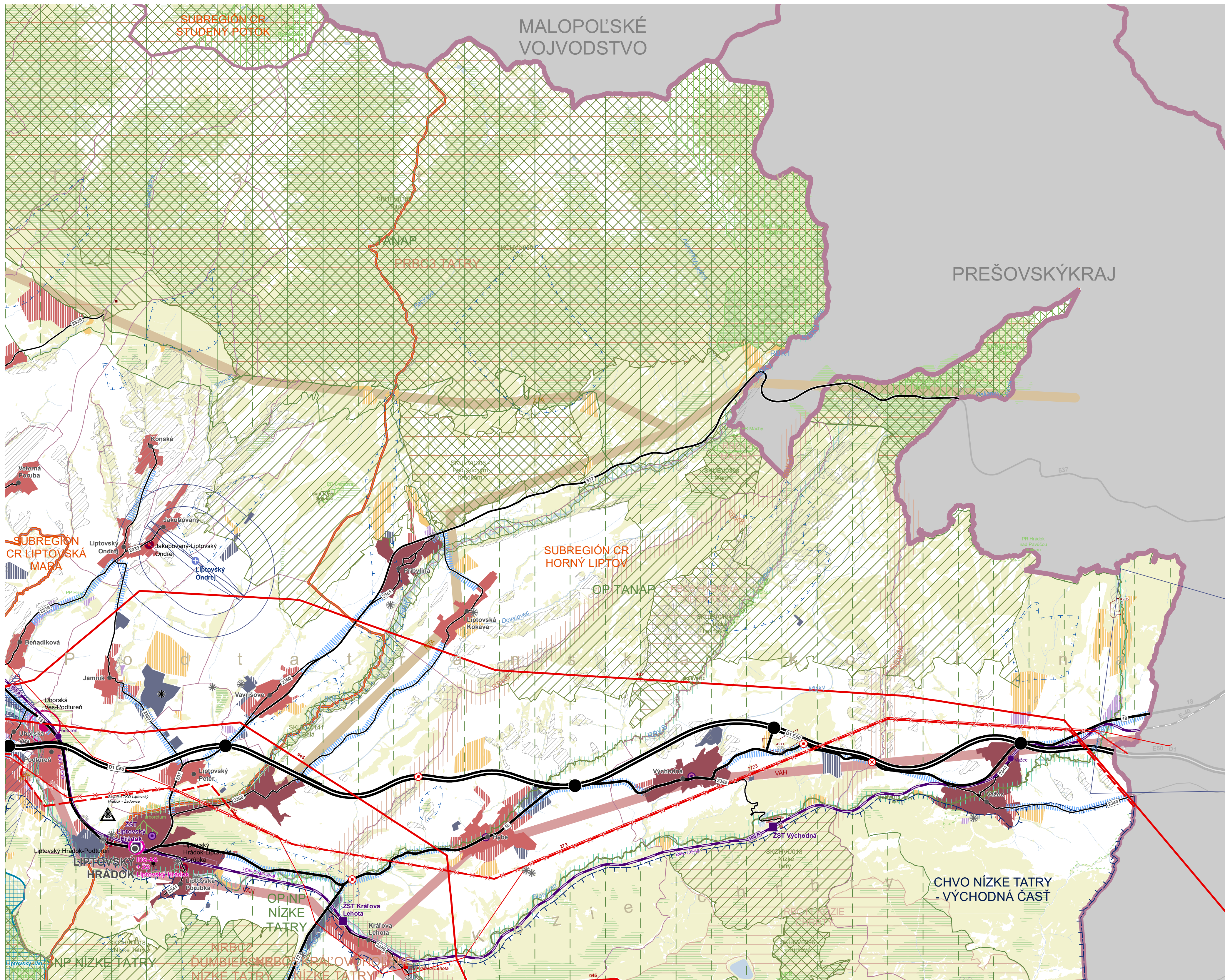
ÚZEMNÝ PLÁN REGIÓNU ŽILINSKÉHO KRAJA - KONCEPT - VARIANT 1 KOMPLEXNÝ VÝKRES PRIESTOROVÉHO USPORIADANIA A FUNKČNÉHO VYUŽÍVANIA ÚZEMIA
