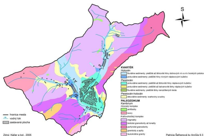
Obrázok 3 Geologická stavba mesta Revúca
