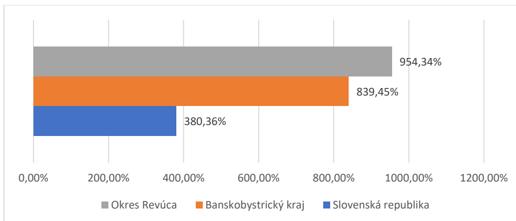
Graf 87 Tuhé emisie – produkcia v tonách, porovnanie rokov 2010 a 2019
