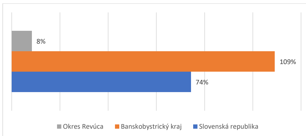
Graf 89 Oxid dusíka – produkcia v tonách, porovnanie rokov 2010 a 2019
