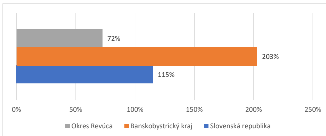
Graf 90 Oxid uhoľnatý – produkcia v tonách, porovnanie rokov 2010 a 2019
